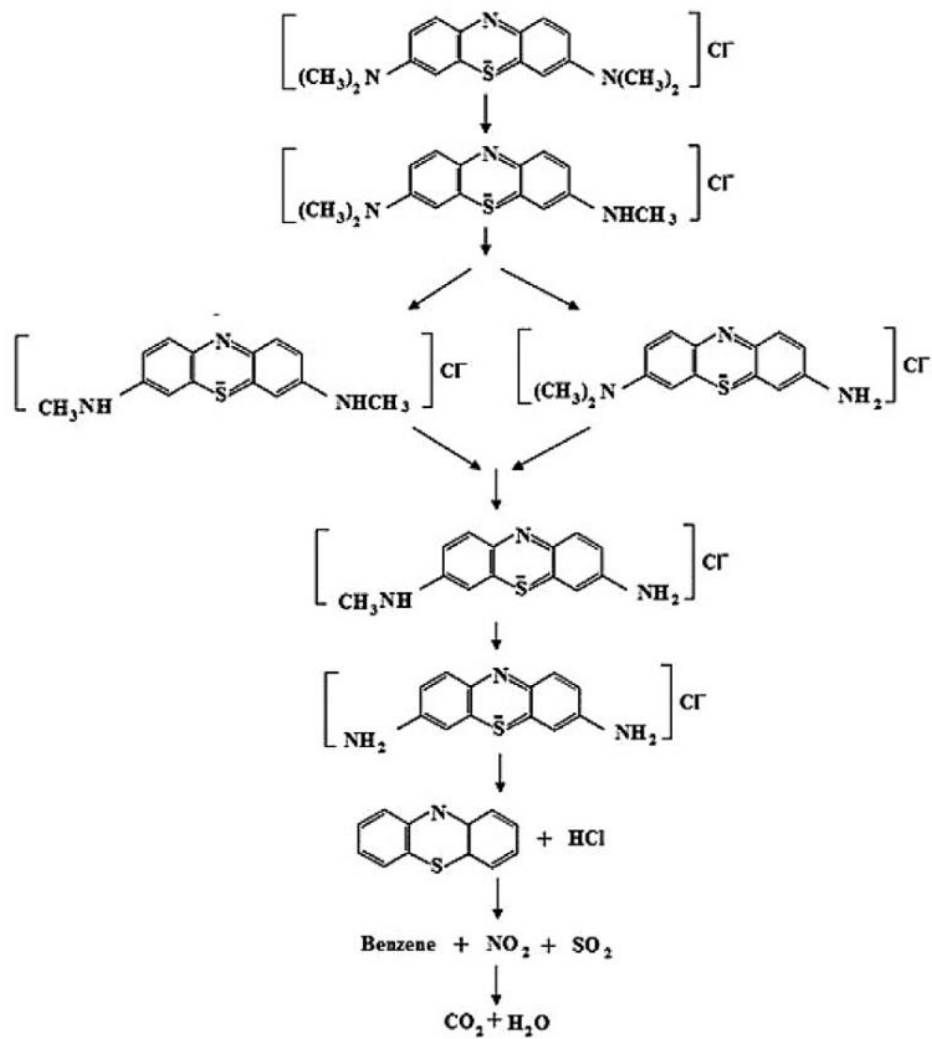
Obr. 23: Reakční schéma fotodegradace methylenové modři 47
