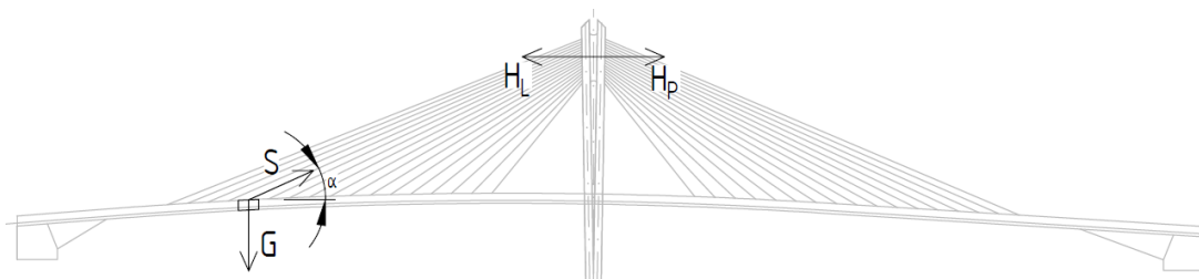
Obrázek 15: Stanovení sil v závěsech
