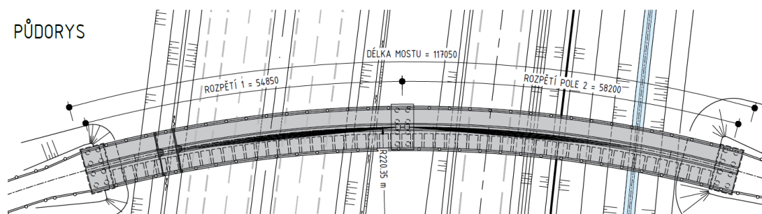
Obrázek 5: Varianta 1 – půdorys
