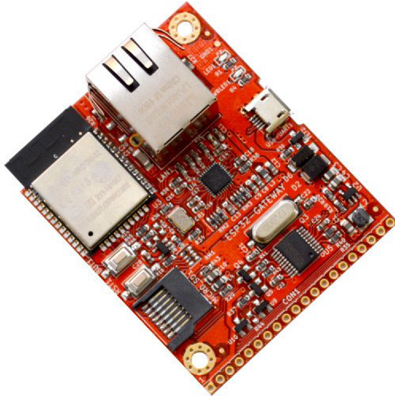
Obr. 5.1: Vývojová deska ESP32-GATEWAY.[13]
