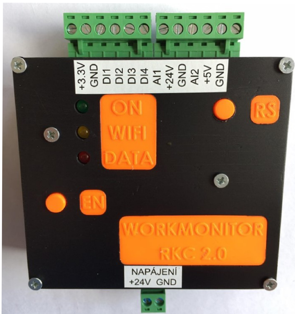
Obr. C.4: Fotografie zařízení s ESP32.
