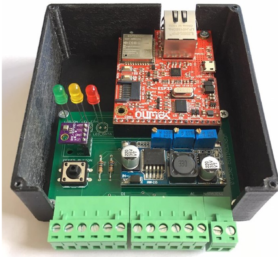
Obr. C.1: Fotografie zařízení s Olimex ESP32-GATEWAY (uvnitř krabičky).
