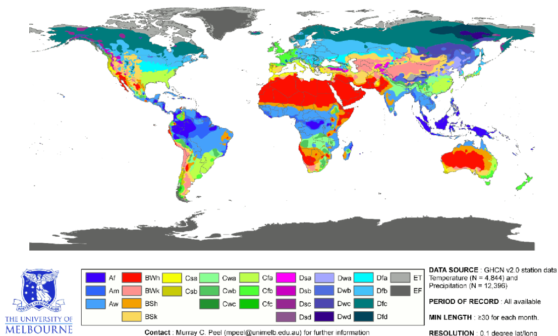
Obrázek 1: Schématické znázornění teplotního klima světa podle Köppena systému, kde je stanoveno 5 hlavních klimatických pásem s 11 základními klimatickými typy. Klimatická pásma jsou značena velkými písmeny: A (tropy), B (aridní podnebí), C (mírné podnebí), D (boreální podnebí), E (studené podnebí). Zdroj: Peel et al., 2007.
