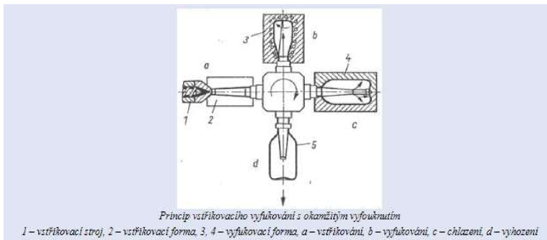
Obr. 2 Princip vstřikovacího vyfukování s okamžitým vyfouknutím [18]
