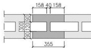
Obrázek 5 - Zjednodušený řez vylehčenou deskou
