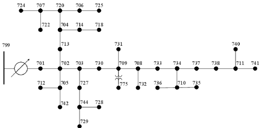
Obrázek 4.5 Rozložení modelu IEEE 37 [12]
