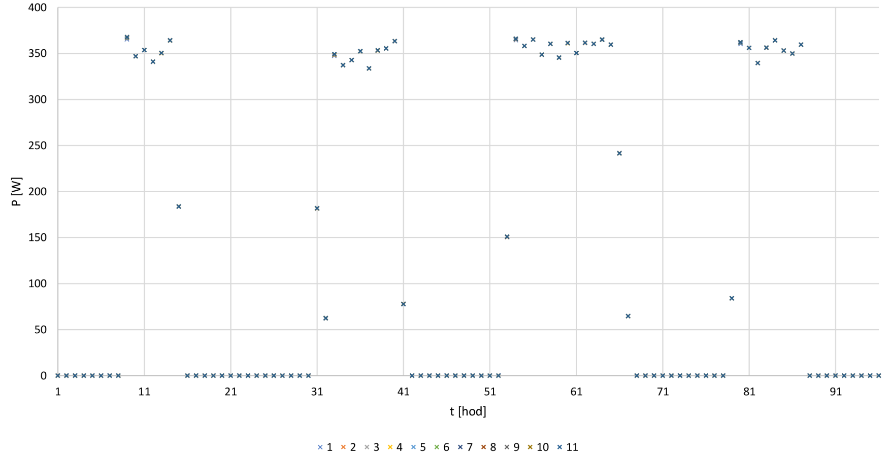
Výkon fotovoltaických elektráren během 96 hodin
