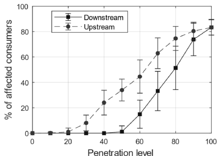
Obrázek 3.4 Podíl odběratelů energie, kteří by měli problém s kvalitou elektřiny v závislosti na penetraci fotovoltaiky [6]
