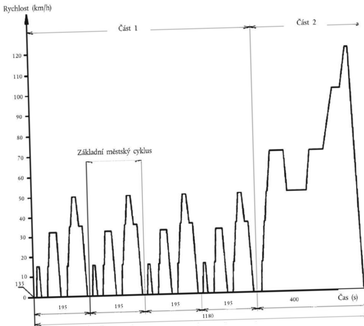
Obr. 2 Grafické znázornění zkoušky typu I – NEDC cyklus [6]
