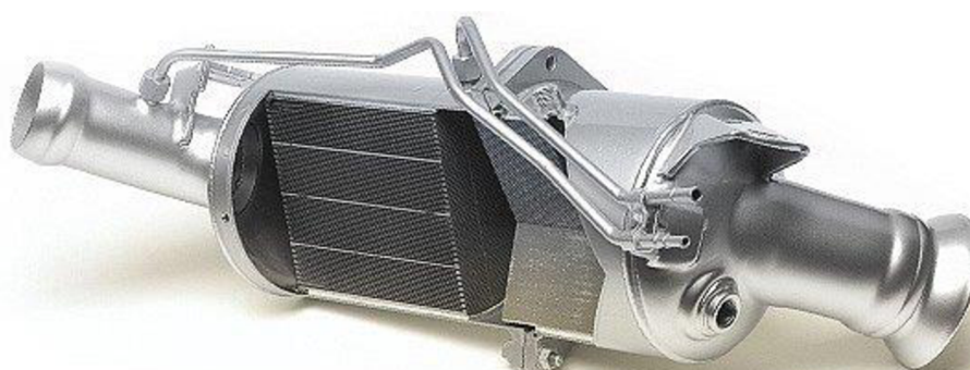
Obr. 7 Průřez DPF filtrem [12]
