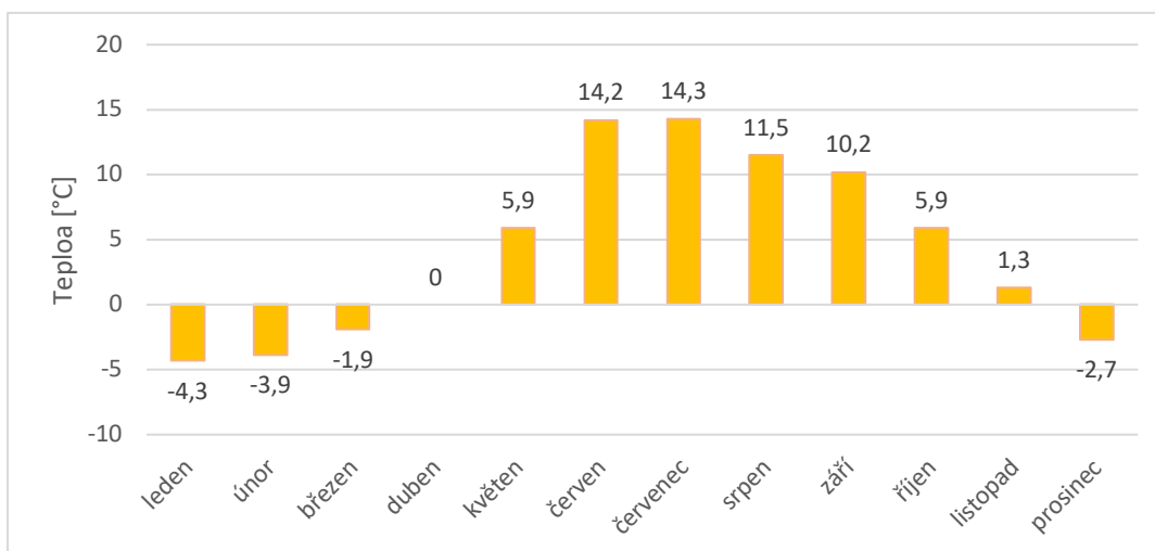
Graf 4 Průměrné měsíční teploty v roce 2021
