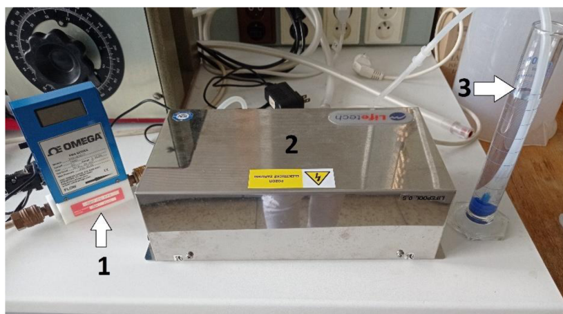
Obrázok 8. Systém prebublania produktov dielektrického bariérového výboja (DBD) do vody, kde č.1 sú prietokomery, č.2 je ozonizátor a č.3 je odmerný valec, v ktorom prebieha prebublávanie produktov do vody
