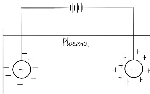
Obrázok 1. Debeyove tienenie[3]
