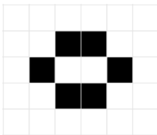
Obrázek 2.2: Stabilní forma Behive . Obrazec v každé generaci má stejný vzor.
