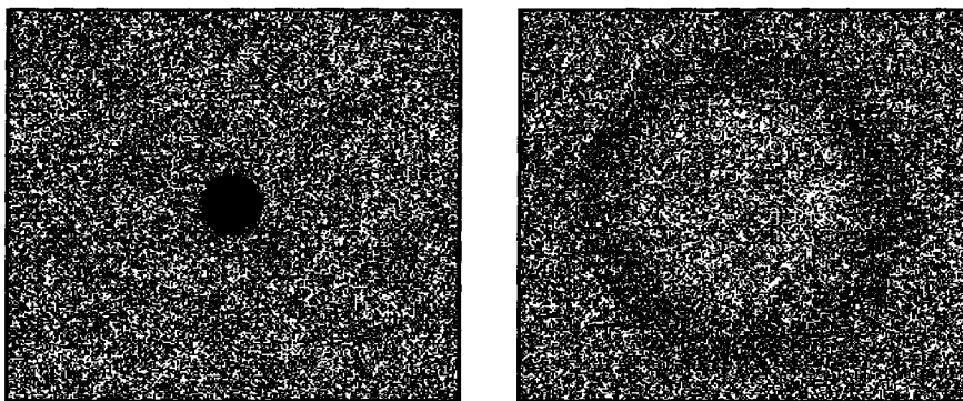
Obrázek 2.15: Ukázka LGCA [11], který využívá HPP model. Na počátku (levý obrázek) je velká koncentrace částic ve středu obrázku. Na pravém obrázku je zobrazena simulace v pokročilém stádiu.
