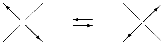
Obrázek 2.17: Grafické znázornění pravidel HPP modelu [41], kde šipka určuje vektor momentu částice. Pozice obsazené částicí jsou znázorněny pomocí šipky, prázdné pozice jsou zobrazeny jako tenká čára.
