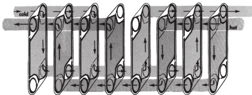
Obr. 12: Viacpriechodové usporiadanie [38]
