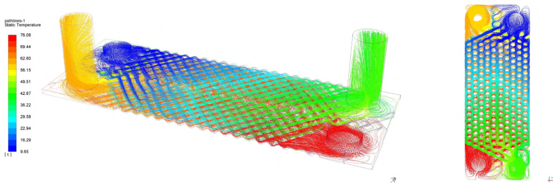
Obr. 75: Prúdnice teplôt pre symetrický dizajn s uhlom prelisovania \beta = 25^\circ
