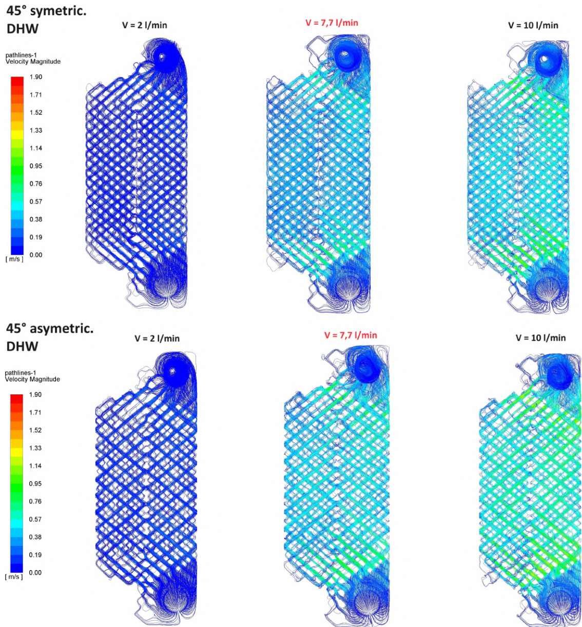
Obr. 73: Prúdnice rýchlosti pre variantu \beta = 45^\circ - DHW strana
