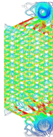
Obr. 70: Prúdnice rýchlosti pre variantu \beta = 25^\circ - HW strana
