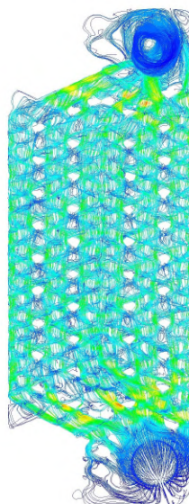
Obr. 70: Prúdnice rýchlosti pre variantu \beta = 25^\circ - HW strana
