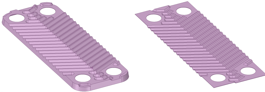
Obr. 43: Úprava dosky výmenníka pre numerickú simuláciu
