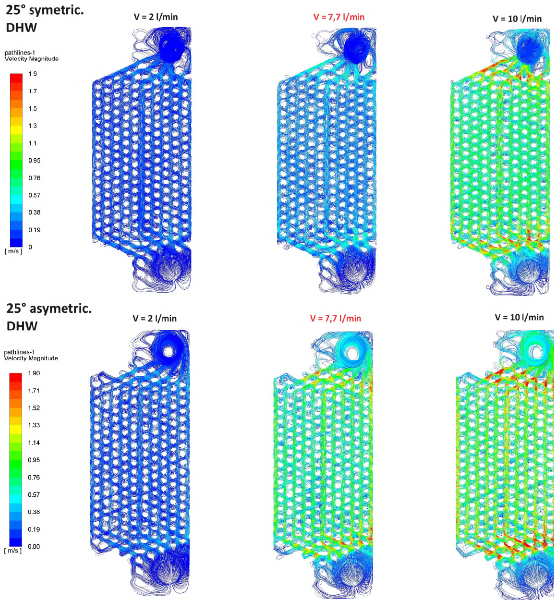
Obr. 72: Prúdnice rýchlosti pre variantu \beta = 25^\circ - DHW strana
