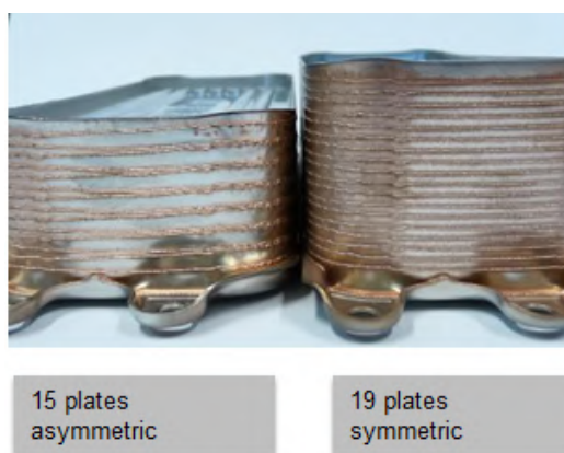
Obr. 17: Porovnanie asymetrického a symetrického výmenníka pri rovnakom výkone [34]
