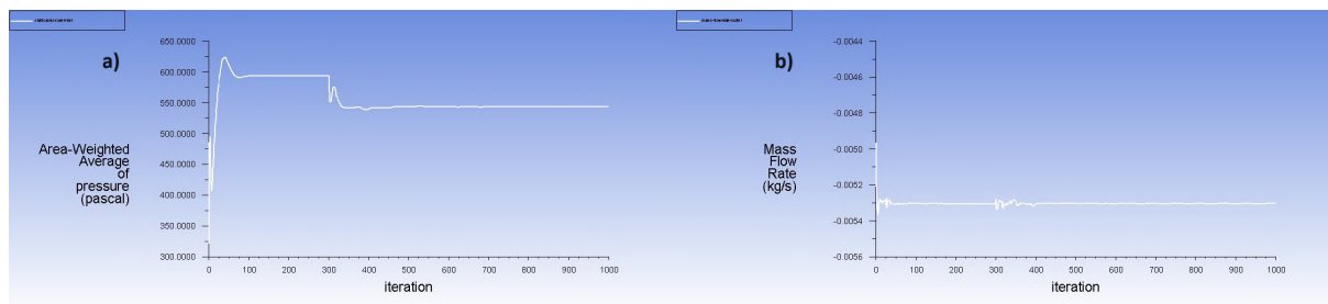
Obr. 65: Konvergencia sledovaných parametrov - CFD simulácia tlakovej straty pri prietoku 2 l/min
