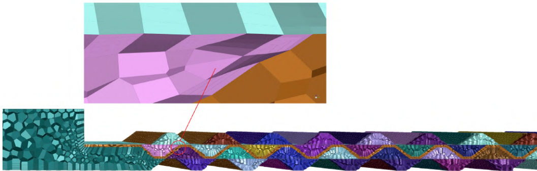
Obr. 49: Objemová sieť pre simuláciu prenosu tepla
