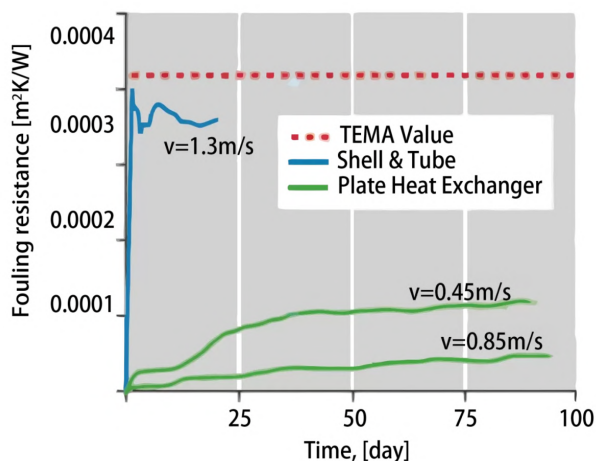
Obr. 29: Závislosť odporu zanášania na čase [16]
