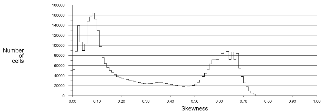
Obr. 53: Histogram (šikmost) - CFD simulácia prenosu tepla
