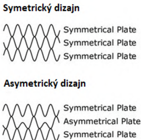
Obr. 18: Konštrukcia symetrického a asymetrického výmenníka tepla [12]
