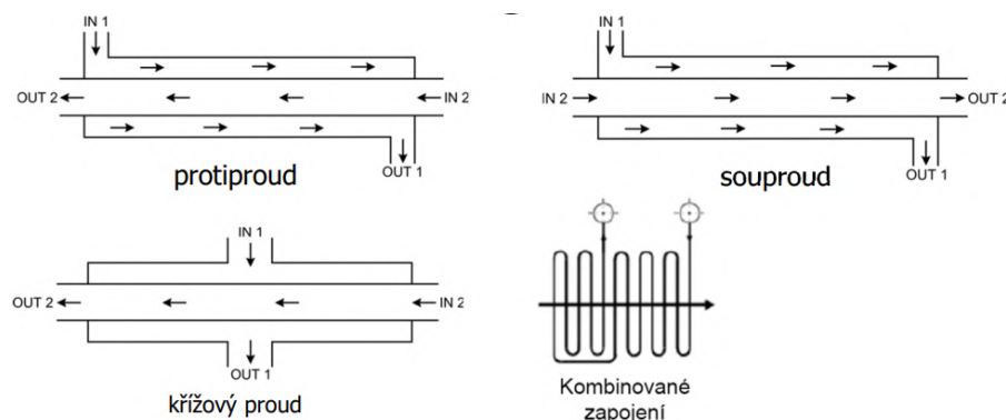
Obr. 2: Rozdelenie typov výmenníkov tepla podľa vzájomného smeru a zmyslu prúdenia [14]
