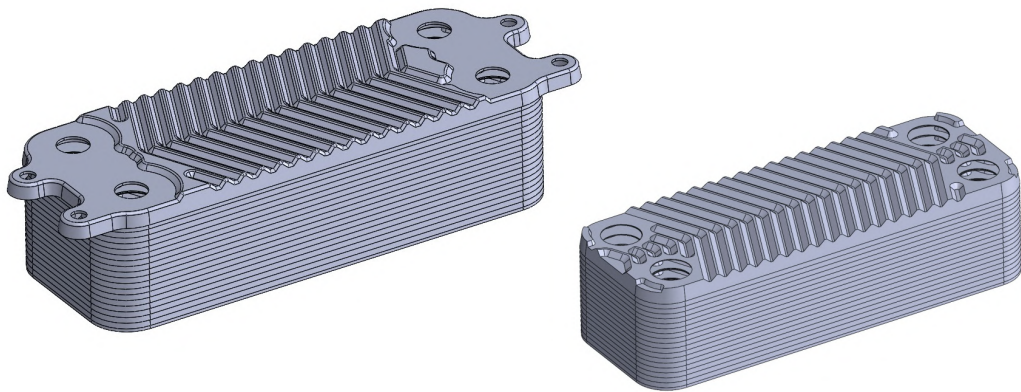
Obr. 42: 3D model doskového výmenníka tepla (uhol prelisovania 25^\circ , symetrický dizajn)
