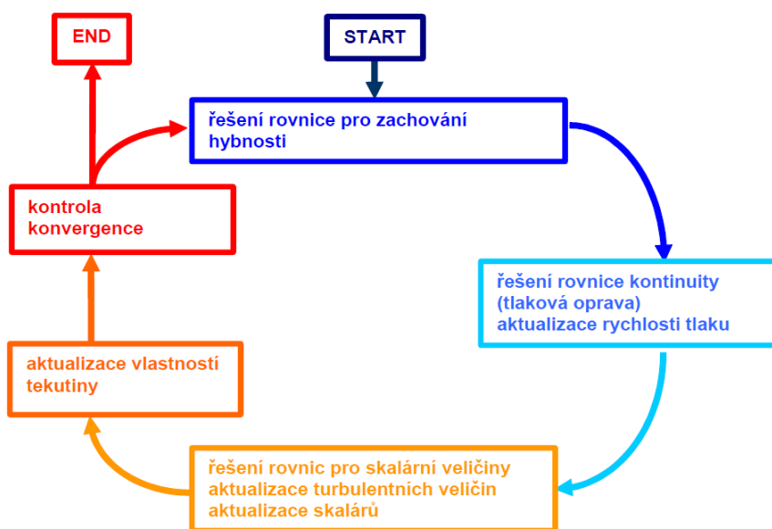
Obr. 54: Diagram algoritmu riešenia Fluentom [23]
