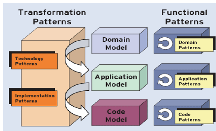
Obr. 2.7: Návrh aplikace MDA [7]
