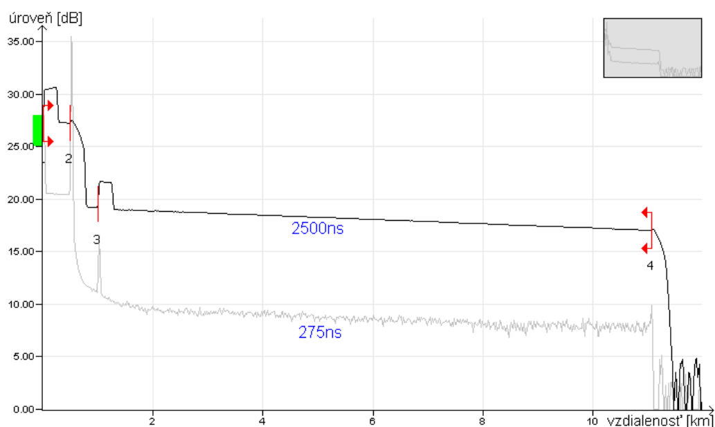
Obr. 9.19: Zmerany graf na vlnovej dĺžke 1625nm pri rôznych pulzoch
