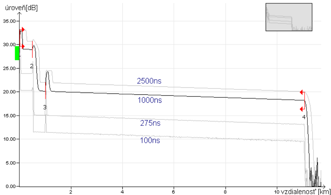
Obr. 9.16: Zmerany graf na vlnovej dĺžke 1550nm pri rôznych pulzoch
