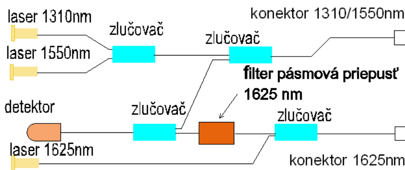
Obr. 9.18: Vnútorne zapojenie prístroja OTDR
