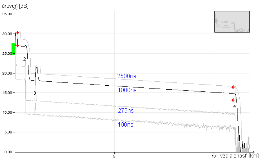
Obr. 9.15: Zmeraný graf na vlnovej dĺžke 1310nm pri rôznych pulzoch
