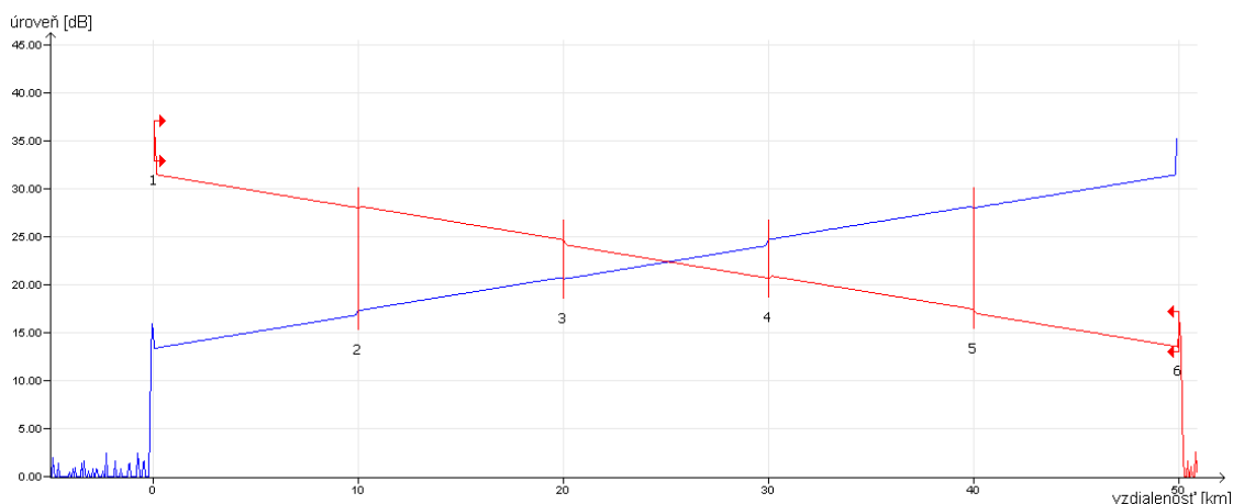
Obr. 9.13: Graf optickéj trasy zobrazený programom Bidir Viewer
