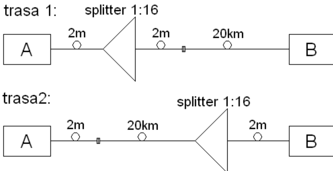
Obr. 10.2: Schémy zapojenia pri meraní prístrojmi FOT-930
