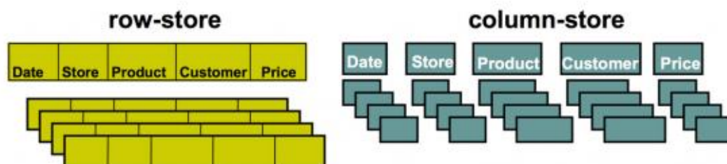
Obrázek 3: Porovnání sloupcové a relační databáze. Zdroj: (MPP & Columnar Databases, 2021)
