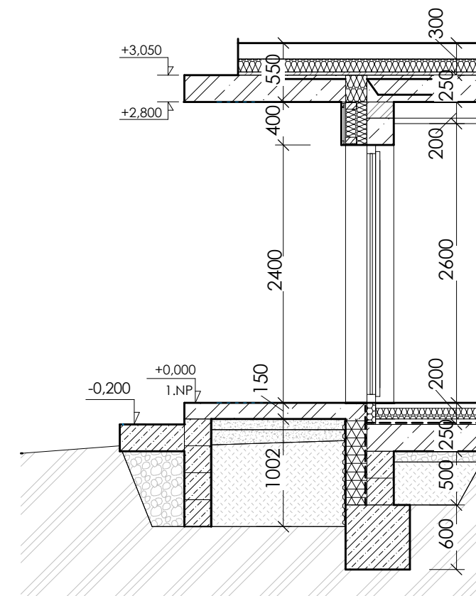
Řez fasádou obytné části 1:50
