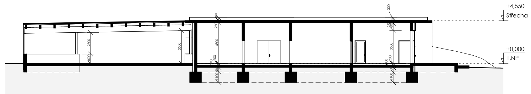
Řez A-A'
