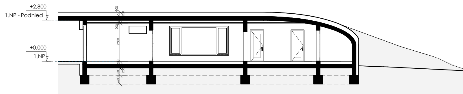
Řez B-B'
