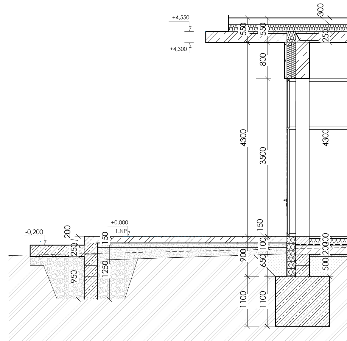
Řez fasádou výrobní části 1:50
