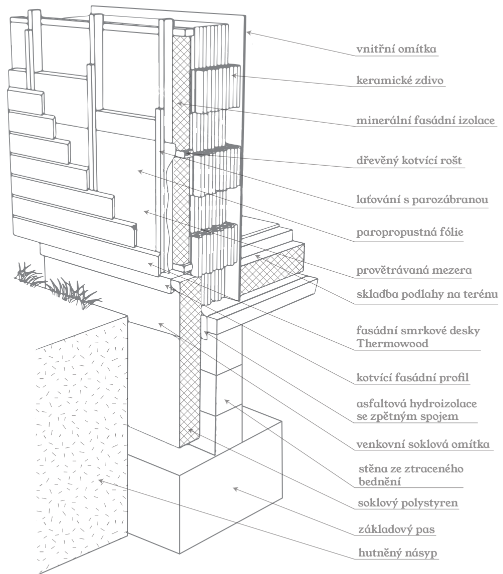
schéma 12:
