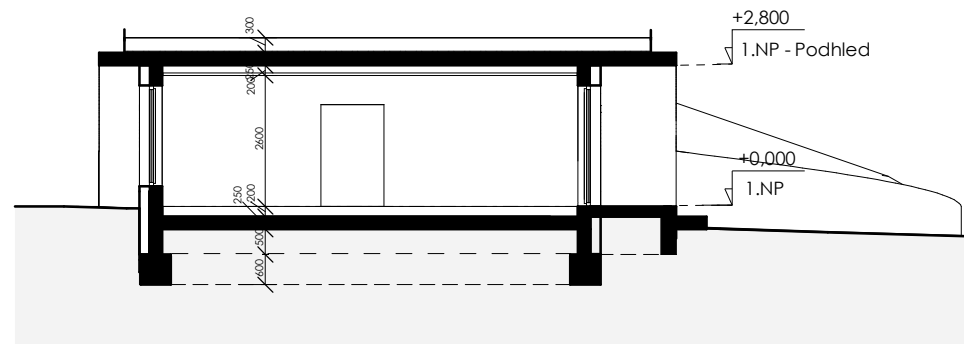
Řez A-A'
