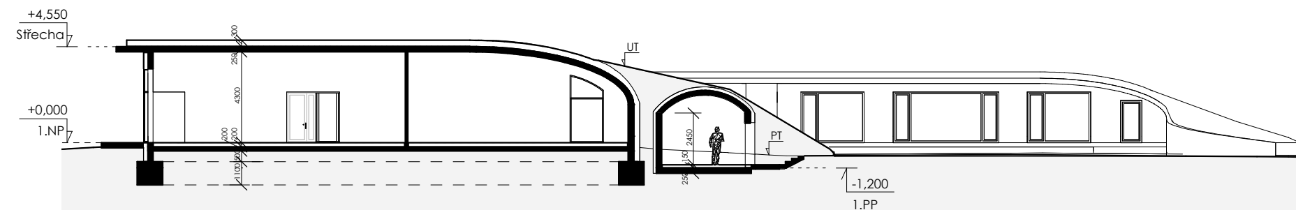
Řez B-B'
