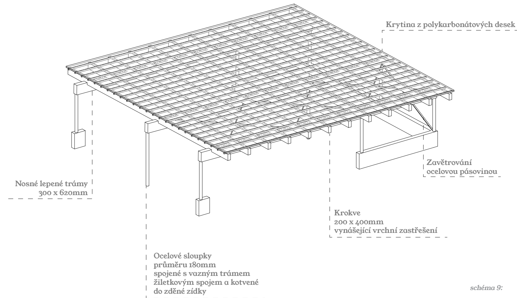
schéma 9: konstrukční schéma dřevěné rámové konstrukce
