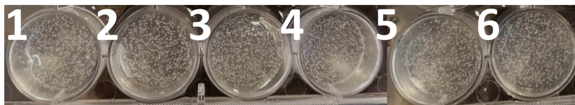
Obrázek 37: Sítování alginátu uhličitánem vápenatým v kombinaci s GDL – vliv přidavku dihydrogenfosforečnanu draselného.
