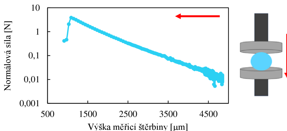
Obrázek 13: Squeeze test s měřicí geometrií o průměru 8 μm.
