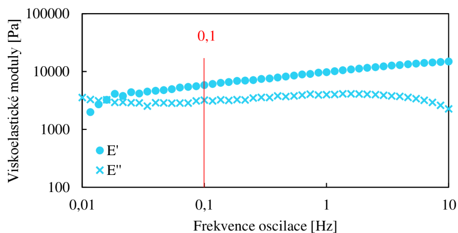
Obrázek 11: Frekvenční test s deformací v tlaku – amplituda deformace 1 %.
