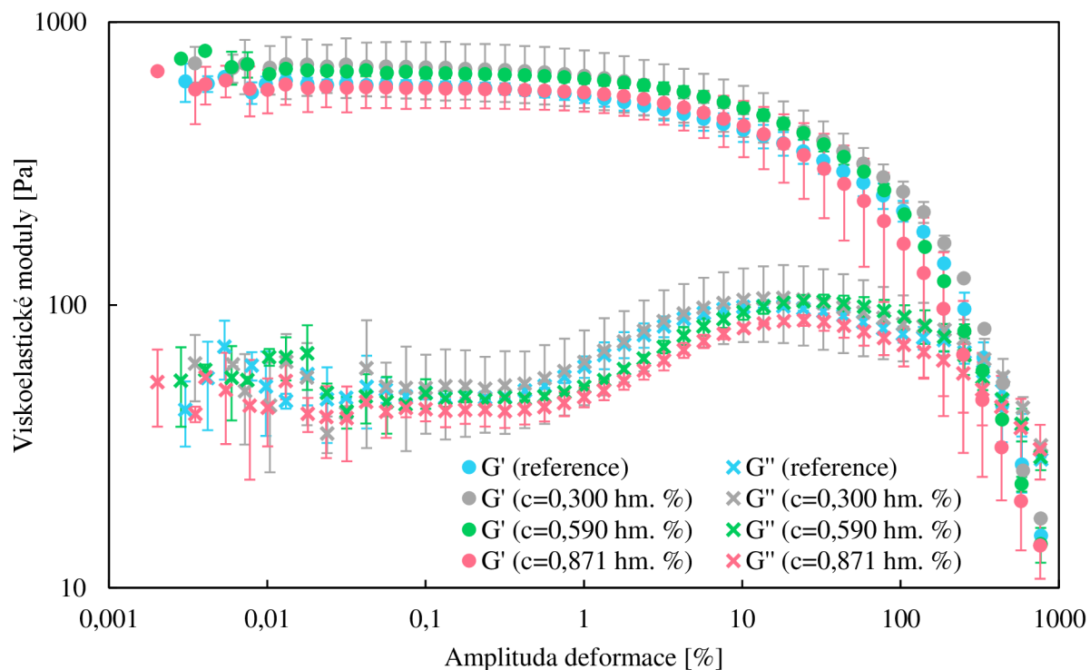
Obrázek 40: Výsledky amplitudových testů s deformací ve smyku – zesíťovaný alginát s přidavkem kyseliny citronové.
