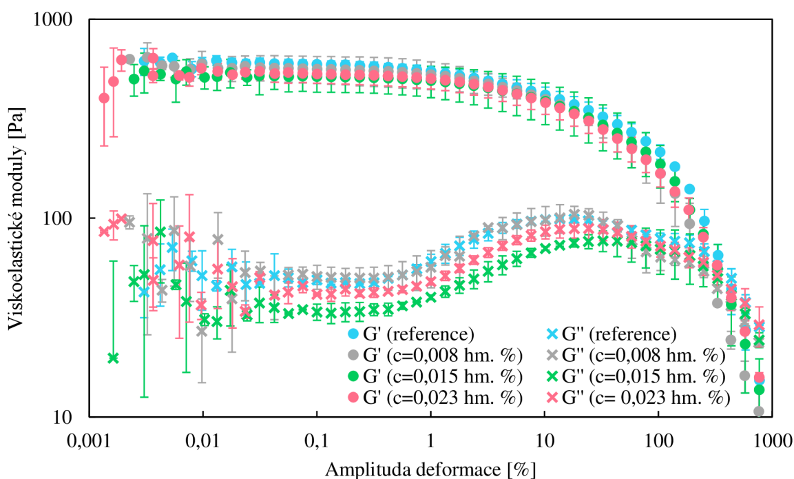
Obrázek 38: Výsledky amplitudových testů s deformací ve smyku – zesíťovaný alginát s přidavkem dihydrogenfosforečnanu draselného.
