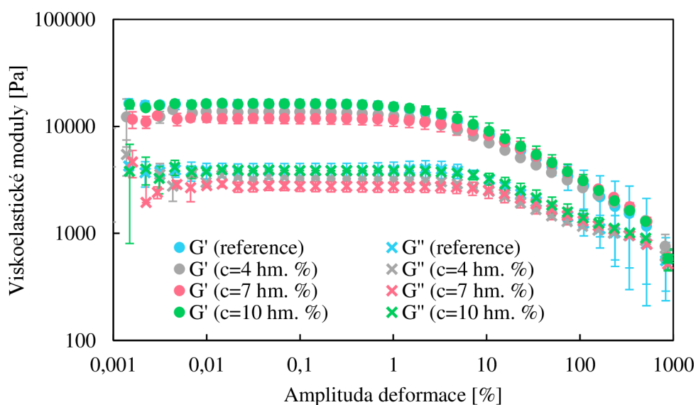
Obrázek 34: Výsledky amplitudových testů s deformací ve smyku – vliv přidavku sacharózy.
