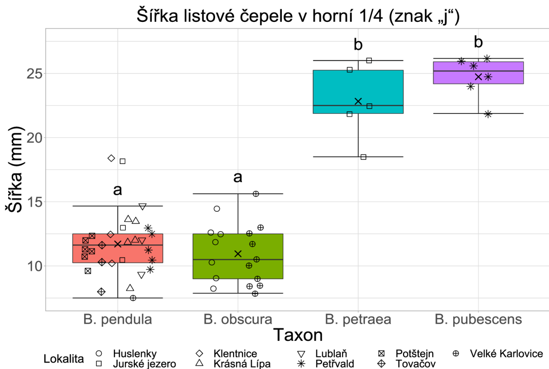
Obr. 20: Krabicový graf porovnávající šířku listové čepele v horní 1/4 mezi taxony a místy odběrů. Šířka listové čepele v horní 1/4 byla pro jednotlivé taxony stanovena jako medián (příčná čára uvnitř krabice) a aritmetický průměr (křížek uvnitř krabice) naměřených hodnot. Body v grafu představují výsledky měření hodnocených jedinců a jsou rozmístěny náhodně, aby nedošlo k jejich vzájemnému překryvu. Místa odběrů jsou rozlišeny příslušnými geometrickými tvary jednotlivých bodů. Chybové úsečky a konce krabic představují ve vztahu k mediánu percentily po 25 %. Taxony označené odlišnými písmeny se od sebe statisticky průkazně liší na hladině významnosti \alpha = 0,05 .
