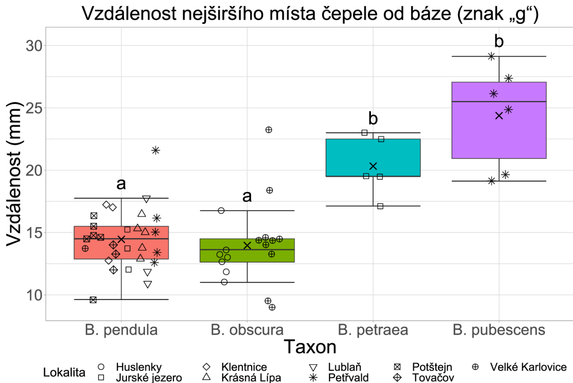
Obr. 19: Krabicový graf porovnávající vzdálenost nejširšího místa čepule od báze mezi taxony a místy odběrů. Vzdálenost nejširšího místa čepule od báze byla pro jednotlivé taxony stanovena jako medián (příčná čára uvnitř krabice) a aritmetický průměr (křížek uvnitř krabice) naměřených hodnot. Body v grafu představují výsledky měření hodnocených jedinců a jsou rozmístěny náhodně, aby nedošlo k jejich vzájemnému překryvu. Místa odběrů jsou rozlišeny příslušnými geometrickými tvary jednotlivých bodů. Chybové úsečky a konce krabic představují ve vztahu k mediánu percentily po 25 %. Taxony označené odlišnými písmeny se od sebe statisticky průkazně liší na hladině významnosti \alpha = 0,05 .
