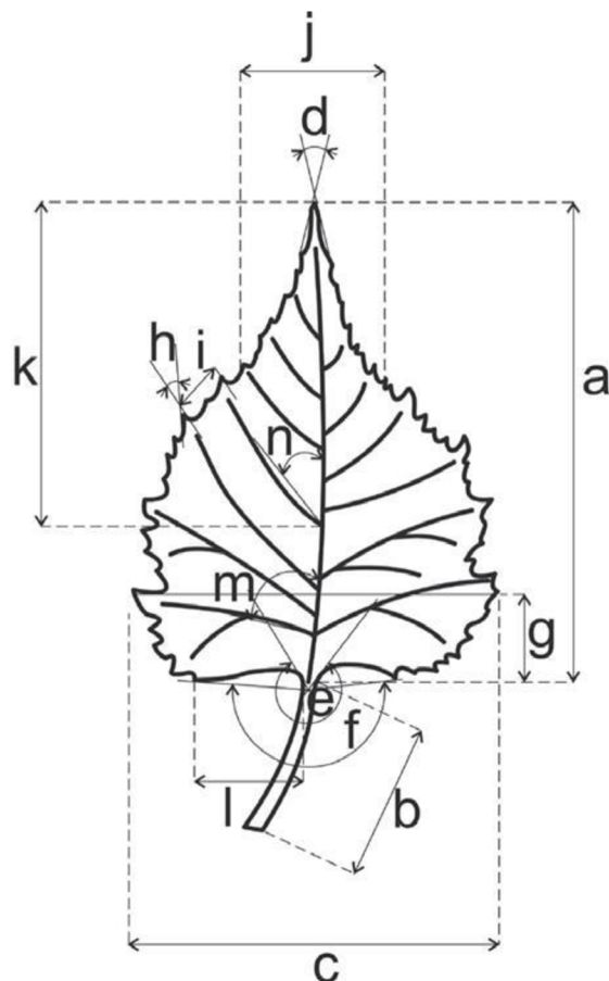
Obr. 13: Grafická ilustrace sledovaných morfologických znaků (a–n). Popis jednotlivých znaků je uveden v Tab. 2. Zdroj: Ešnerová et al. (2012).
