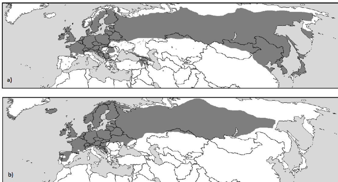
Obr. 11: Areál výskytu břízy bělokoré ( B. pendula ) (a) a břízy pýřité ( B. pubescens ) (b). Zdroj: Dubois et al. (2020).
