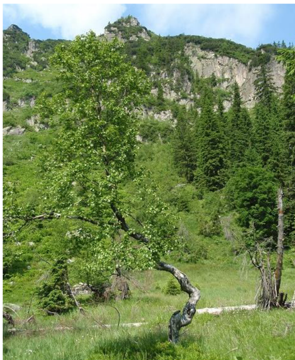
Obr. 6: Bříza karpatská ( B. carpatica ) v Labském dole – záběr na habitus stromu. Zdroj: Ivan Kuneš.
