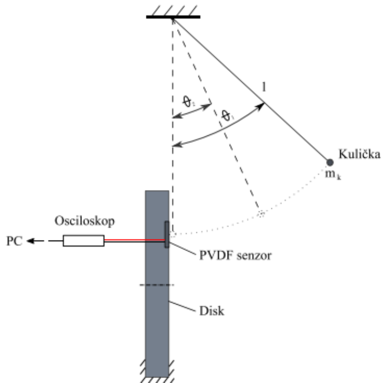
Obrázek 31: Kyvadlová metoda [10]
