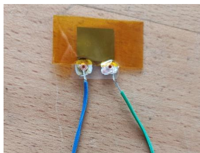
Obrázek 27: Kaptonová izolace
