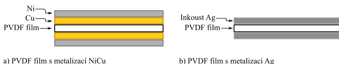
Obrázek 6: Základní typy metalizace: a) CuNi b) Ag
