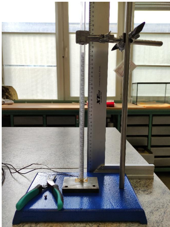
Obrázek 33: Kalibrační trať
