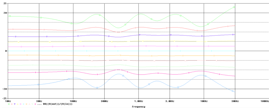
Obr. 22 – Modulová frekvenční charakteristika pětipásmového ekvalizéru – rozmítání všech pásem současně
