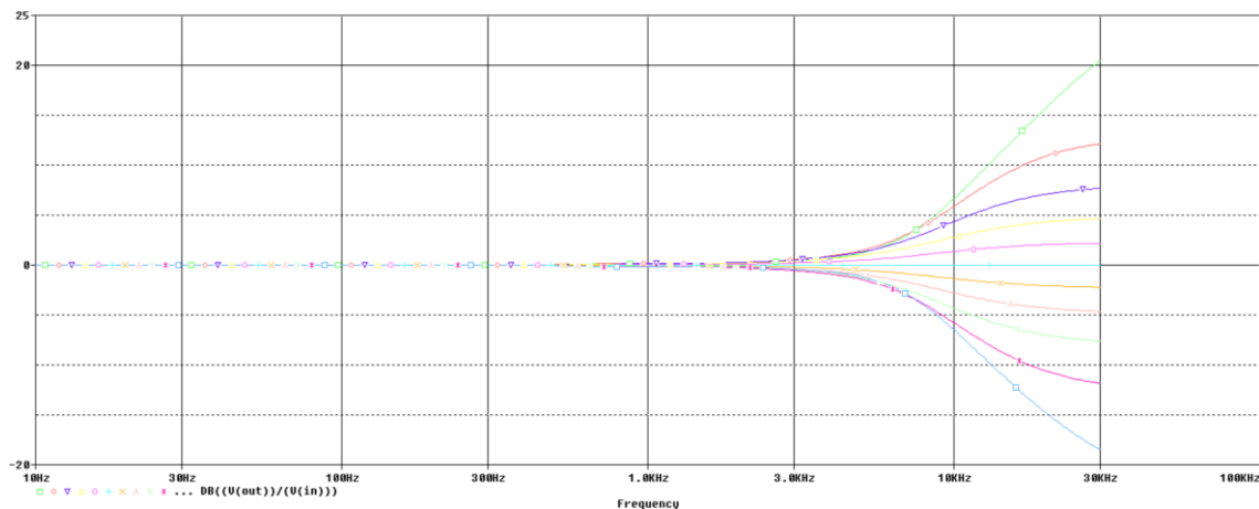
Obr. 21 – Modulová frekvenční charakteristika pětipásmového ekvalizéru s rozmítáním pásma 15 kHz
