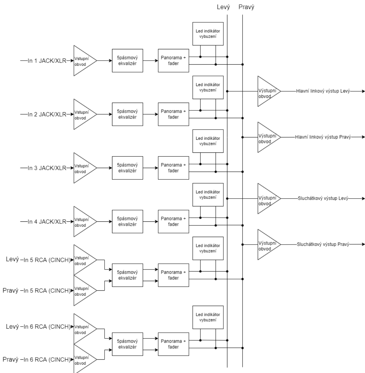
Obr. 1 - Blokové schéma mixážního pultu pro audio signály
