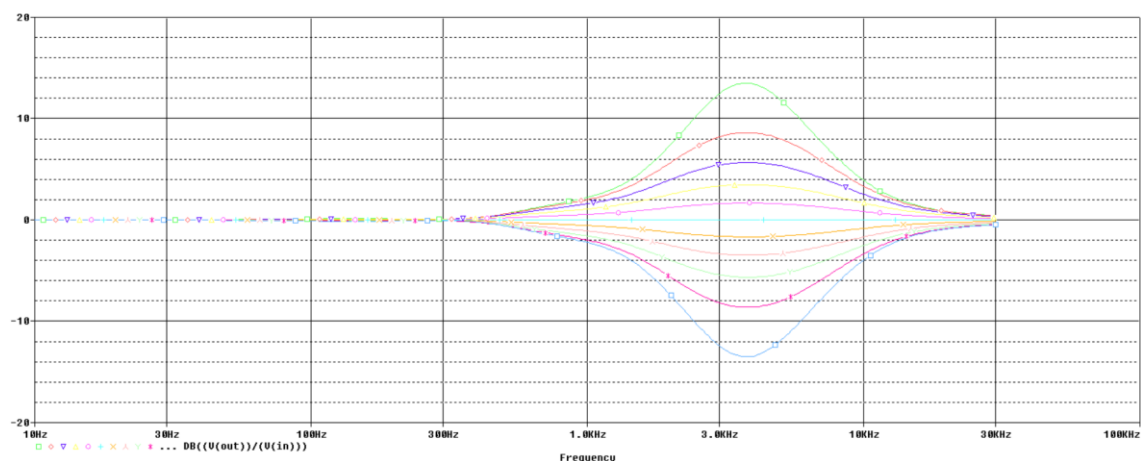
Obr. 20 – Modulová frekvenční charakteristika pětipásmového ekvalizéru s rozmítáním pásma 4 kHz
