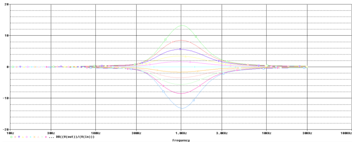
Obr. 19 – Modulová frekvenční charakteristika pětipásmového ekvalizéru s rozmítáním pásma 1 kHz
