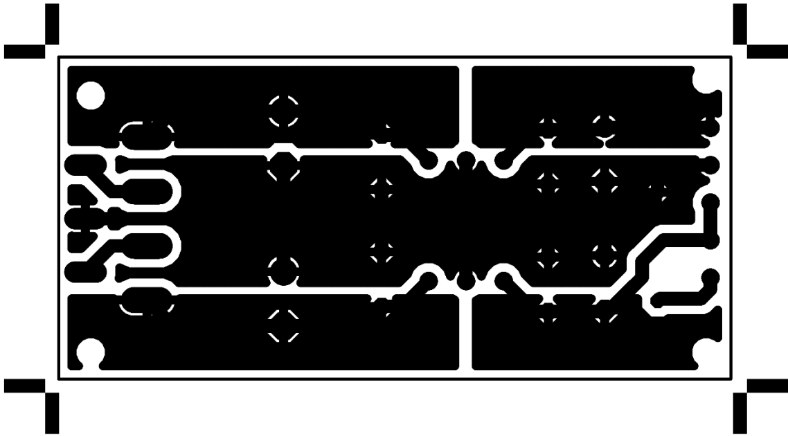
Návrh DPS + osazovací plán – rozměr 63x30 mm, M1:2
