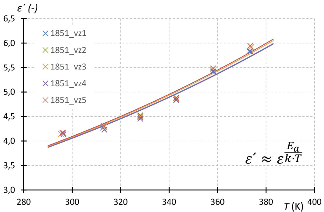
Obr. 17 Závislost relativní permitivity na teplotě pro vzorky sady 1851
