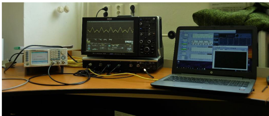
Obrázek 4.17 - Pracoviště použité pro sestavení modulačního signálu
