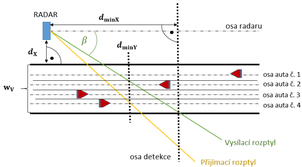
Obrázek 2.2: Půdorys měřicího systému a vliv směrovosti antény v horizontálním směru
