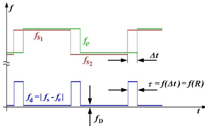
Obrázek 1.17: Princip modulace BFSK (Převzato z [11])
