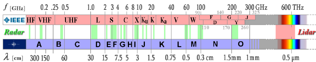
Obrázek 1.2: Frekvenční spektrum elektromagnetického vlnění (Převzato z [4])
