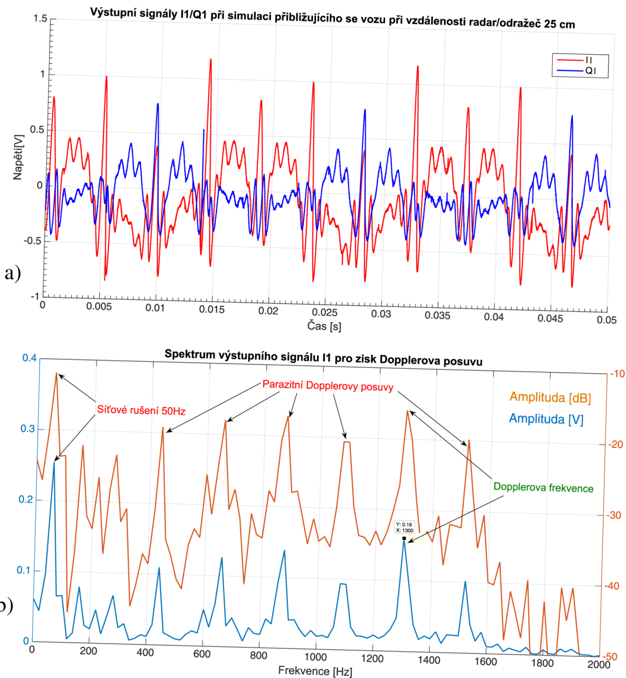
Obrázek 4.12 - Výsledky simulace přibližujícího se vozu pro vzdálenost radar/odražeč 25 cm, Časové průběhy výstupních složek I1/Q1 a) Spektrum výstupního signálu I1 b)
