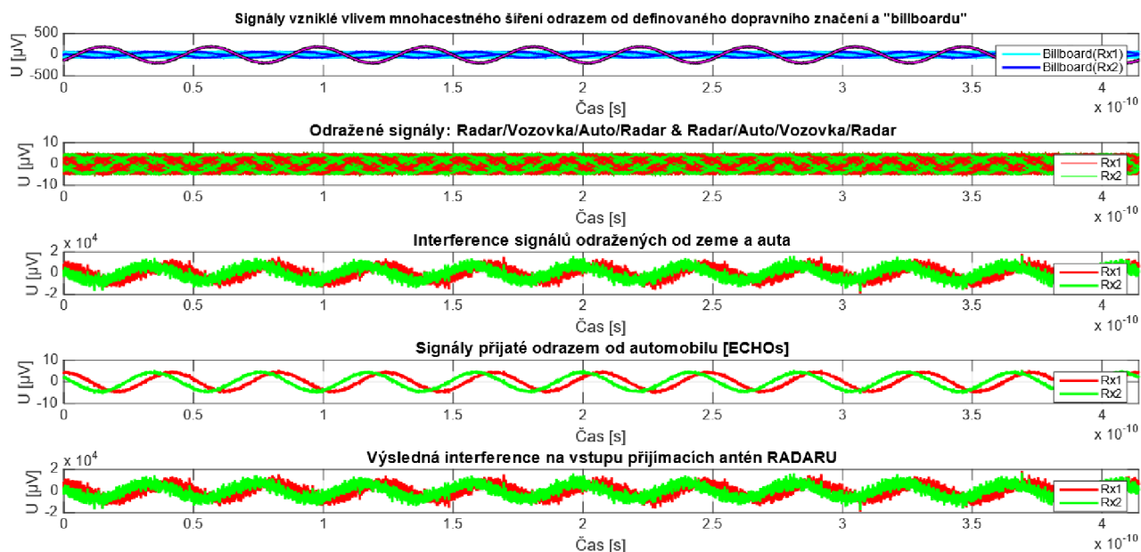
Obrázek 3.18: Konstruktivní interference, kde postupně Shora – Paprsky značené zeleně a žlutě, Červeně, Jejich interference, Užitečný signál odražený od automobilu, Interference všech signálů (dole)
