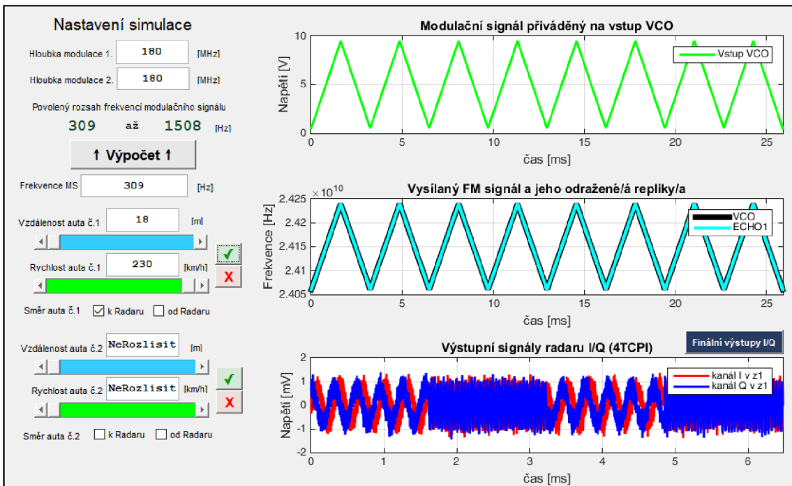
Obrázek 3.42 - Oprava na Obrázek 3.41 ilustrovaného efektu dle vzorce 1/(T_{CP\text{min}} - t_{d\text{min}}) uvedeného v podkapitole 3.5 (Stejný simulovaný případ jako na Obrázek 3.41)
