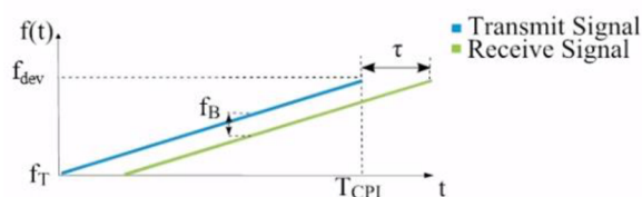
Obrázek 1.11: Proces frekvenční modulace pro měření statického objektu (Převzato z [9])
