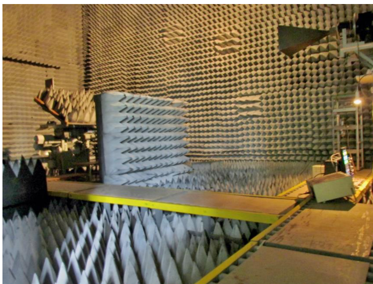
Obrázek 4.19 - EMC komora
