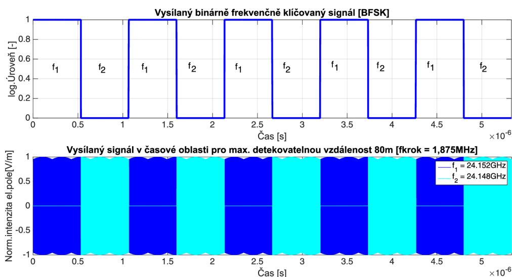
Obrázek 3.6: Vysílací proces BFSK
