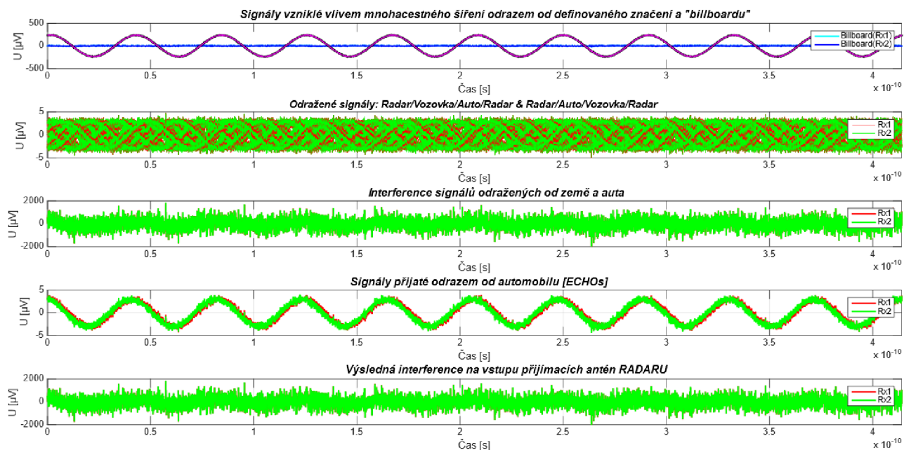
Obrázek 3.17: Destruktivní interference, kde postupně Shora – Paprsky značené zeleně a žlutě, Červeně, Jejich interference, Užitečný signál odražený od automobilu, Interference všech signálů (dole)
