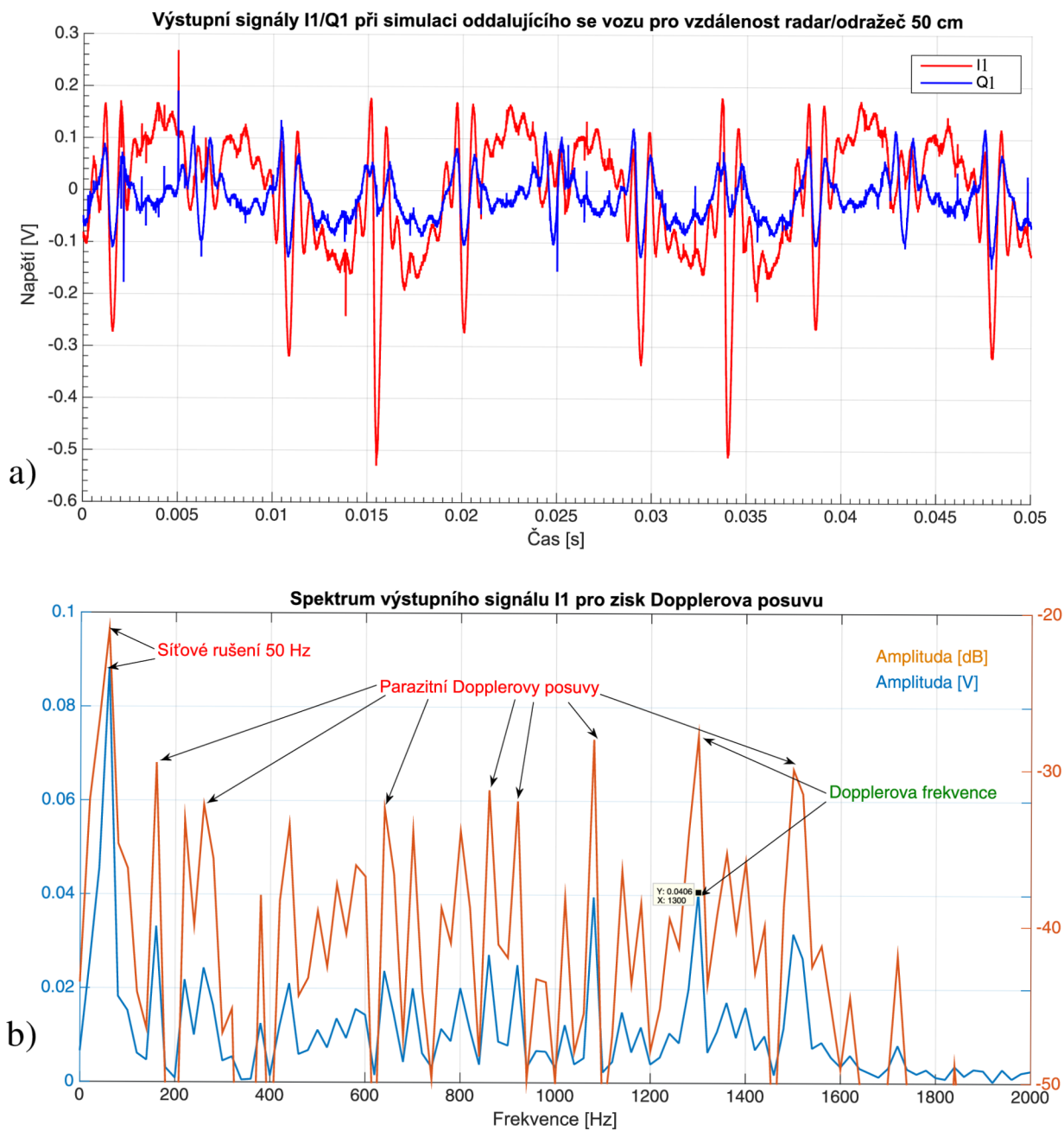
Obrázek 4.13 - Výsledky simulace oddalujícího se vozu pro vzdálenost radar/odražeč 50 cm, Časové průběhy výstupních složek I 1 /Q 1 a) Spektrum výstupního signálu I 1 b)
