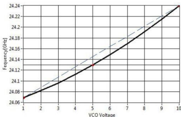
Obrázek 3.22 - Vzájemný vztah mezi frekvenčním a napětovým vyjádřením modulačního signálu
