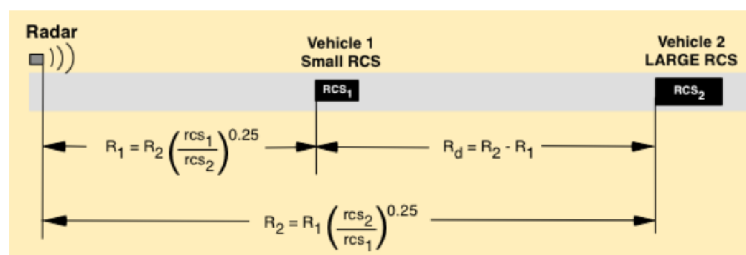
Obrázek 2.16 - Ilustrace pro vysvětlení závislosti velikosti přijatého signálu na RCS automobilu (převzato z [5])
