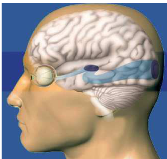
Obr. 2.2 Zrakové ústrojí [8]
