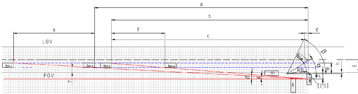
Obr. 4.6 Plánek křižovatky [24]
