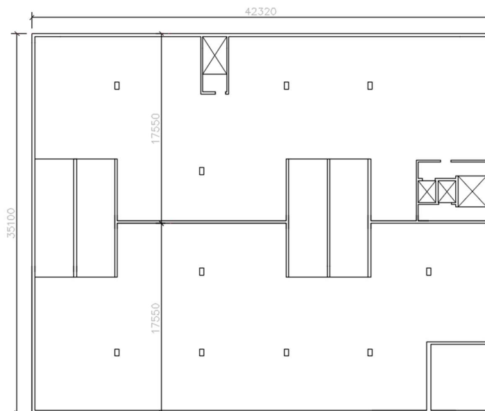
Obrázek 2.2.: Půdorysný pohled na stropní desku 7NP
