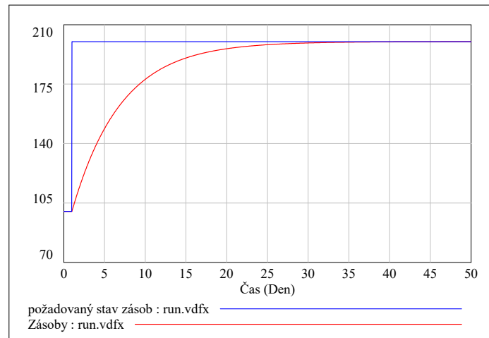
Obrázek 18: Informační zpoždění - simulace
