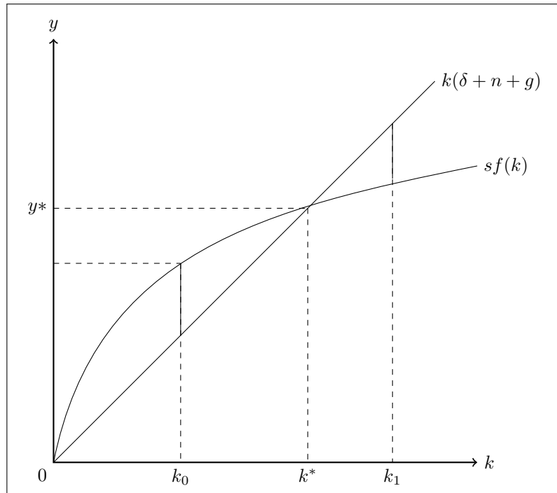
Obrázek 5: Rovnovážný stav v Solow-Swanově modelu s technologickým pokrokem a růstem pracovního kapitálu
