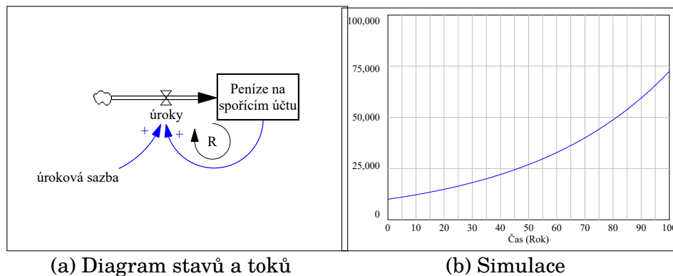
Obrázek 13: Sebepeposilující zpětnovazební smyčka
