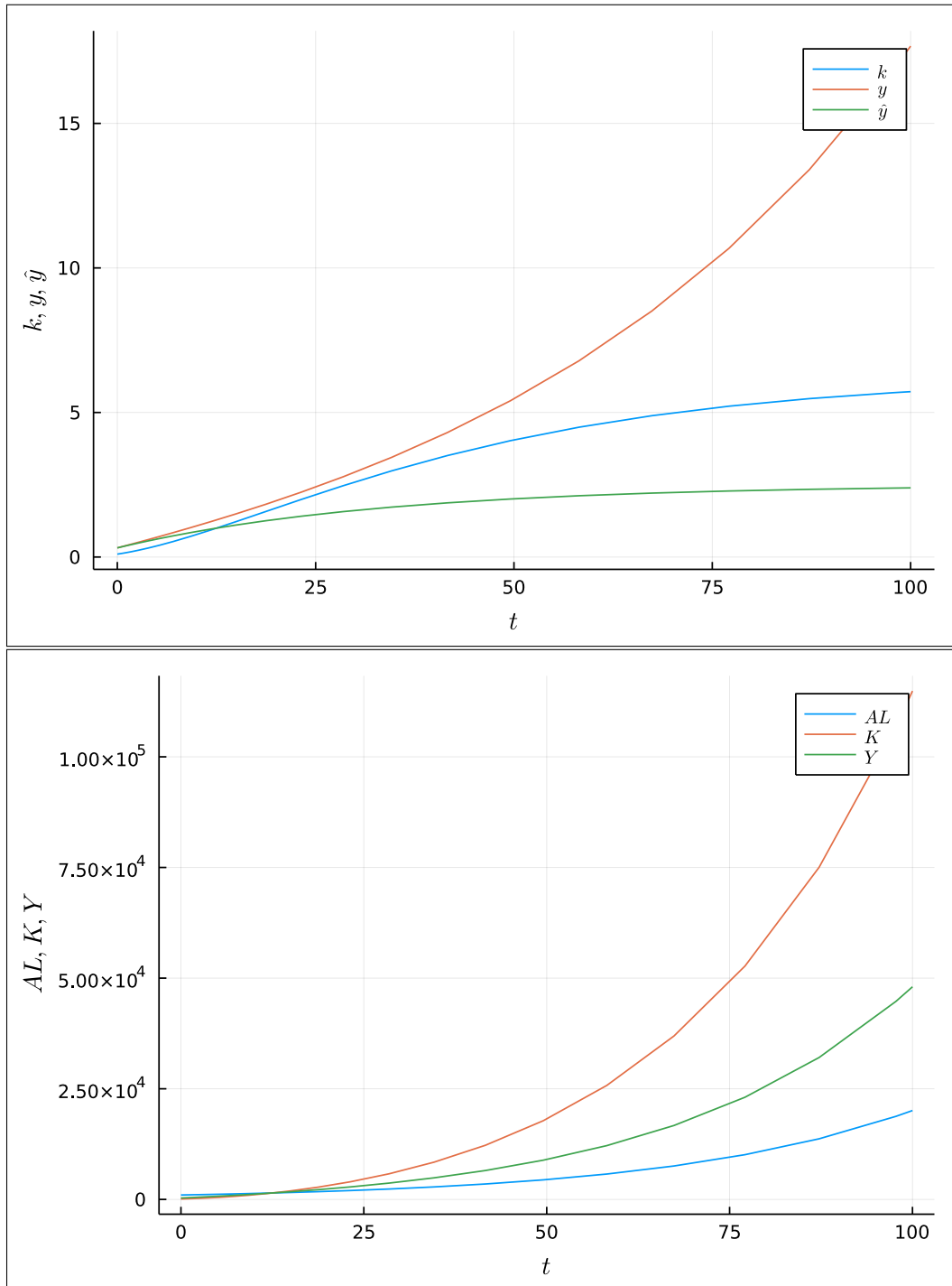
Obrázek 6: Numerická simulace Solow-Swanova modelu
