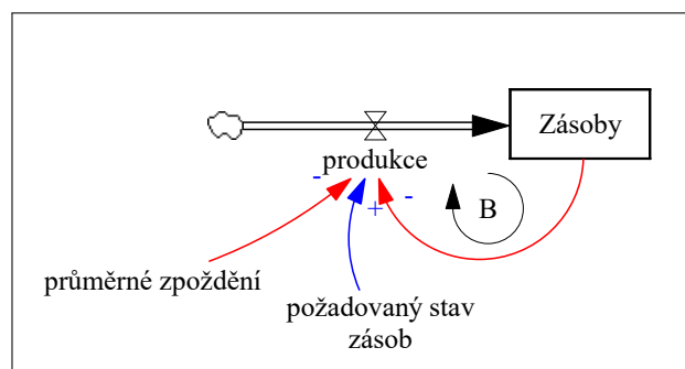
Obrázek 17: Informační zpoždění - diagramové vyjádření
