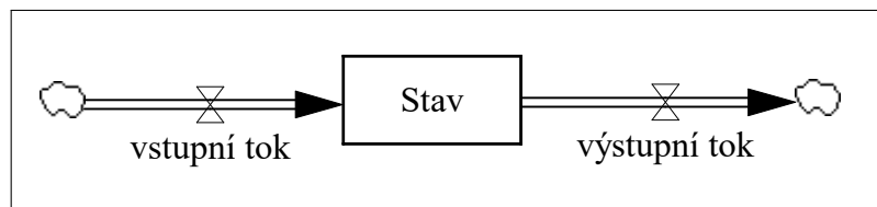
Obrázek 11: Prvky diagramu stavů a toků
