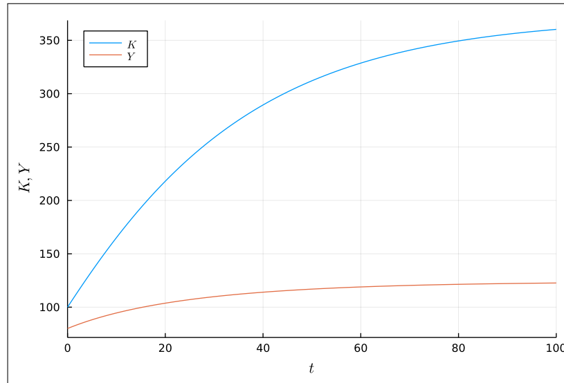
Obrázek 4: Numerická simulace zjednodušeného Solow-Swanova modelu
