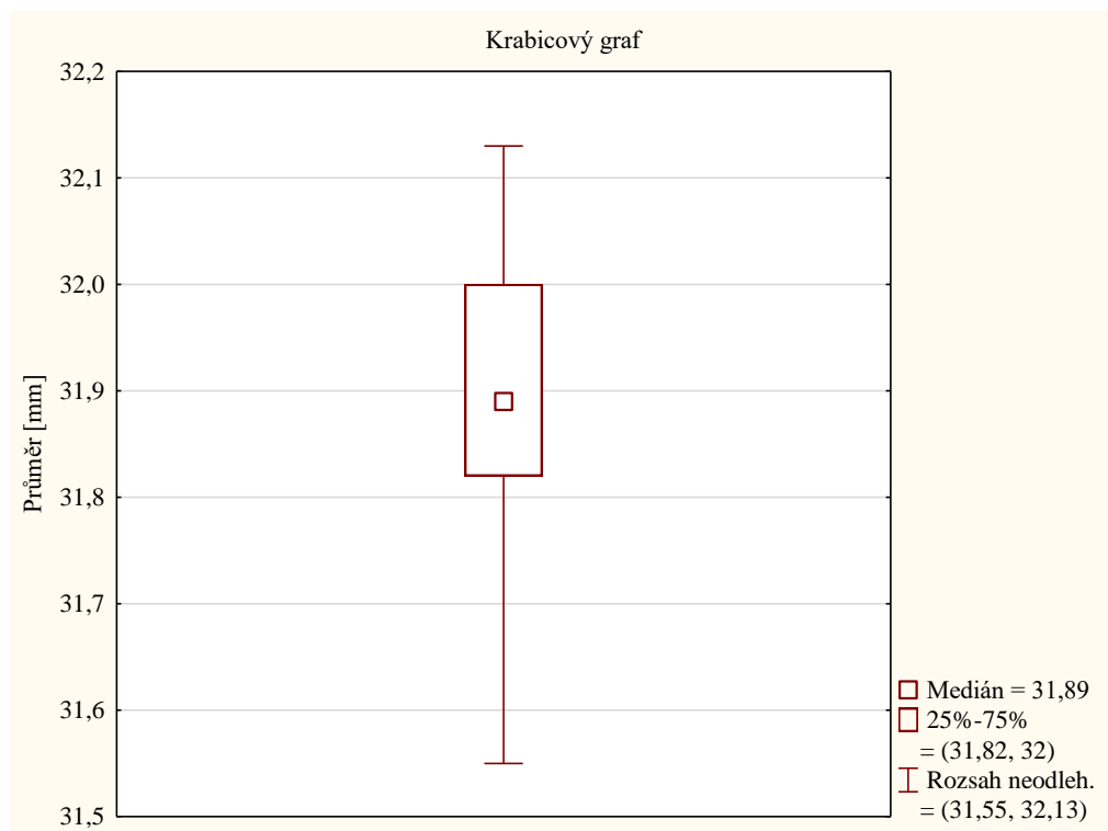
Obrázek 6 - Krabicový graf
