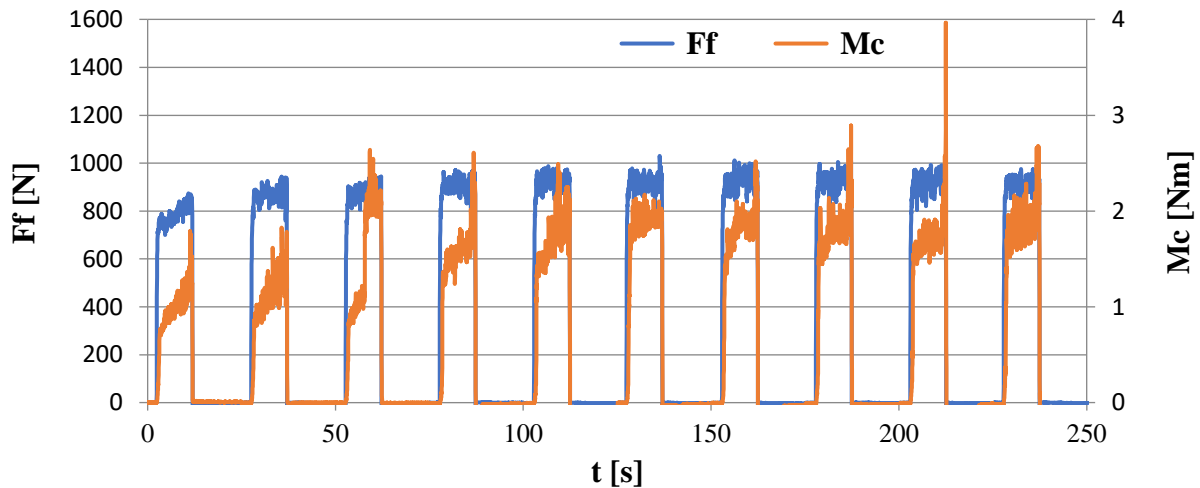
Obr. 15 Graf – vrták A, 0. měření, 10 děr.
