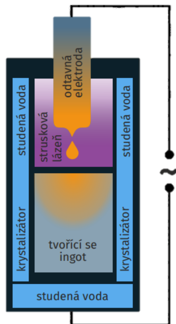
Obr. 6 Schéma elektrostruskového přetavování. [9]
