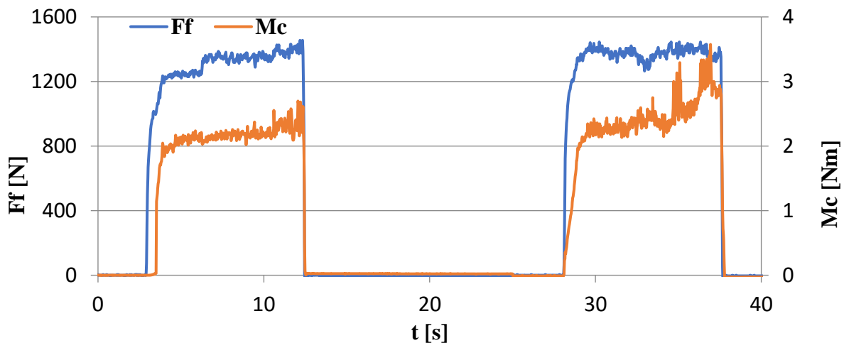
Obr. 20 Graf – vrták B, pružinová ocel, 2. měření, 13 děr.
