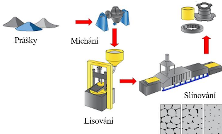
Obr. 7 Prášková metalurgie. [14]
