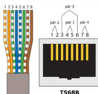
Obrázek 19: Zapojení kabelu dle TIA/EIA T568A a T568B (20)
