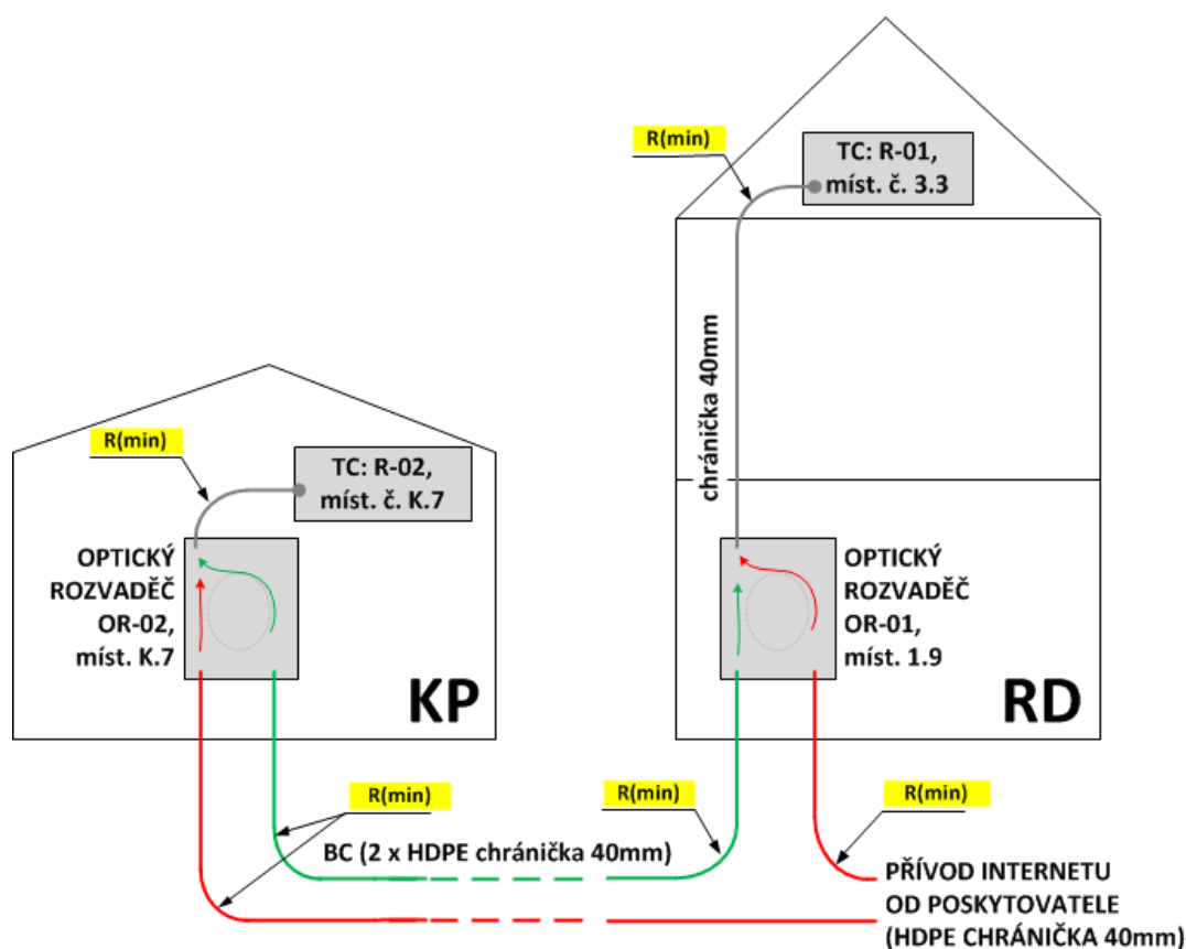
Obrázek 36: Návrh BC a provedení trasy internetového připojení (vlastní zpracování)
