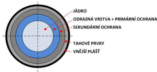
Obrázek 17: Průřez optickým kabelem (18, s. 96)
