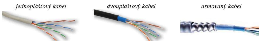
Obrázek 22: Konstrukce plášťů kabelů (20), (21)
