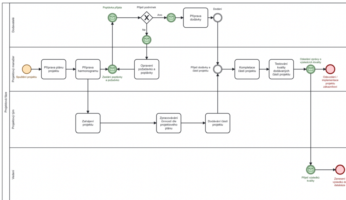
Obrázek 15 Projektová fáze
