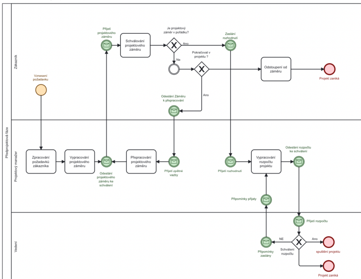
Obrázek 14 Předprojektová fáze
