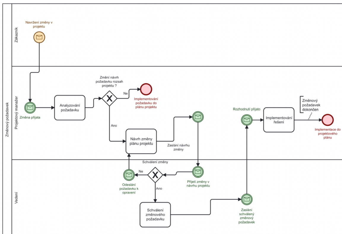
Obrázek 13 Změnový požadavek
