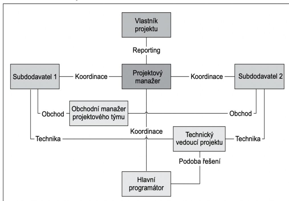
Obrázek 4 Komunikační mapa
