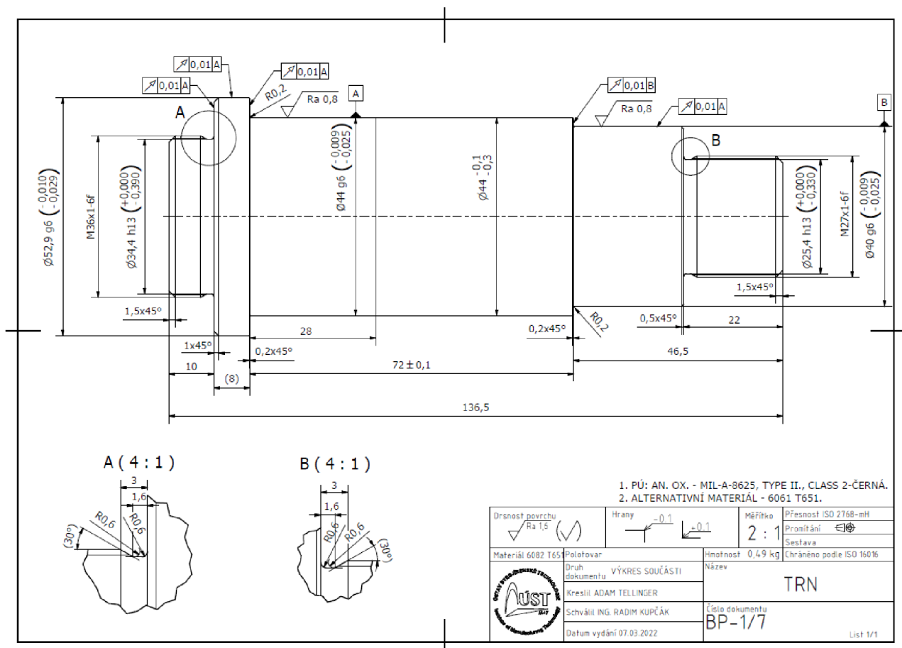
Obr.30 Výkres trnu.
