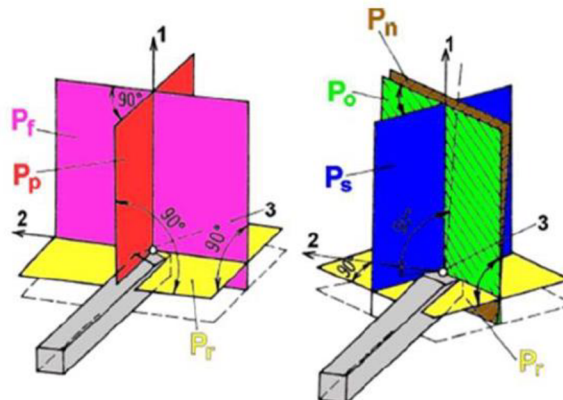
Obr. 22 Nástrojové roviny nože [29].
