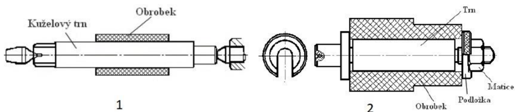
Obr. 9 Kuželový trn (1), válcový trn (2) [7].
