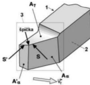
Obr. 21 Části soustružnického nože [29].
