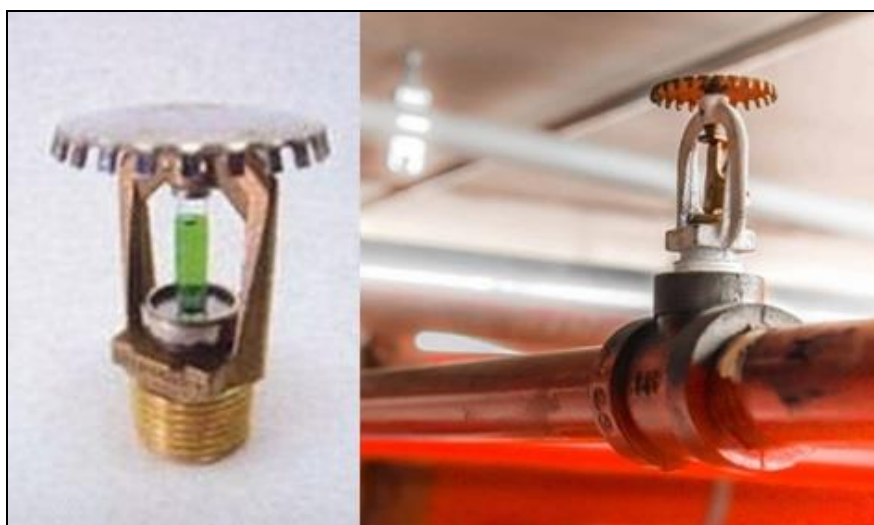
Obrázek 23: Sprinklerová hlavice stojatá
