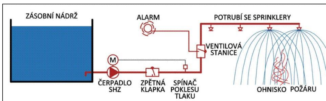
Obrázek 30: Stabilní hasicí zařízení
