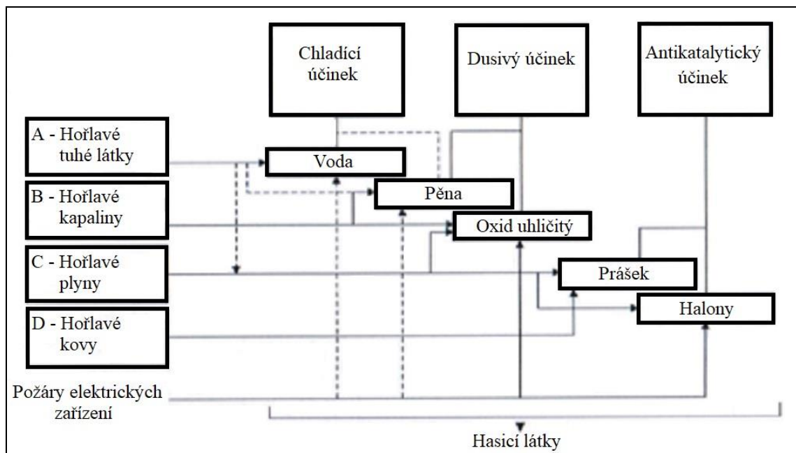
Obrázek 7: Princip hašení
