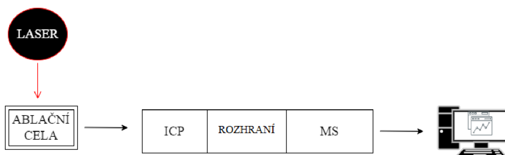
Obrázek 4: Schéma LA-ICP-MS
