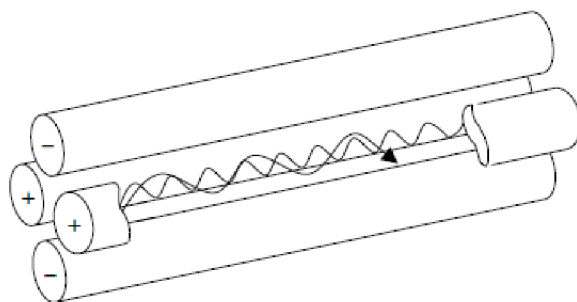
Obrázek 6: Kvadrupólový analyzátor [39]
