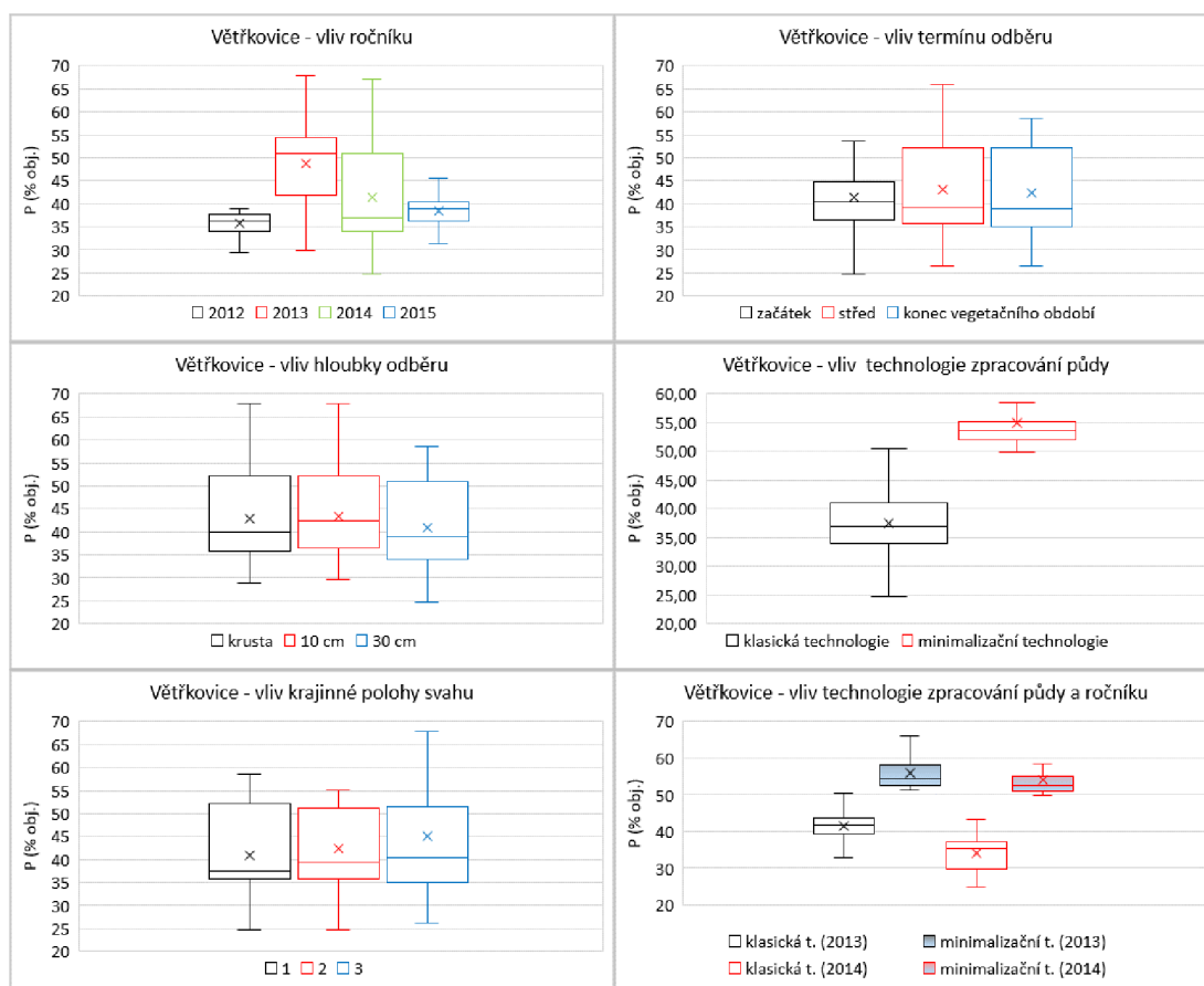
Graf. 5 Průměrné hodnoty pórovitosti v % obj. v lokalitě Větrkovice
