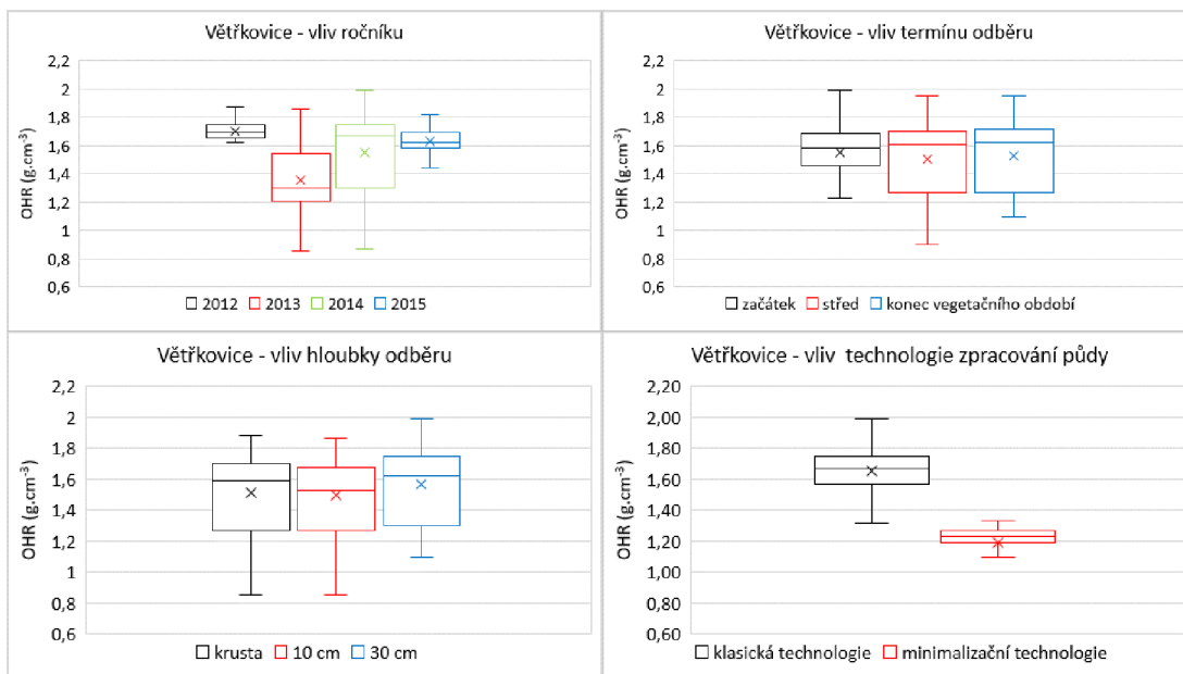
Graf. 1 Průměrné hodnoty obj. hmotnosti redukované v g.cm^{-3} v lokalitě Větrkovice
