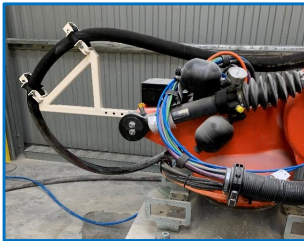
Obrázek 29 - Vedení kabelů a hadic s materiálem
