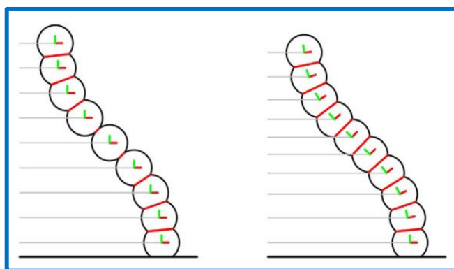
Obrázek 19 - Svislý řez vrstvami se stejnou tloušťkou vrstev běžnou metodou (vlevo) a metodou tangenciální kontinuity (vpravo) [52]
