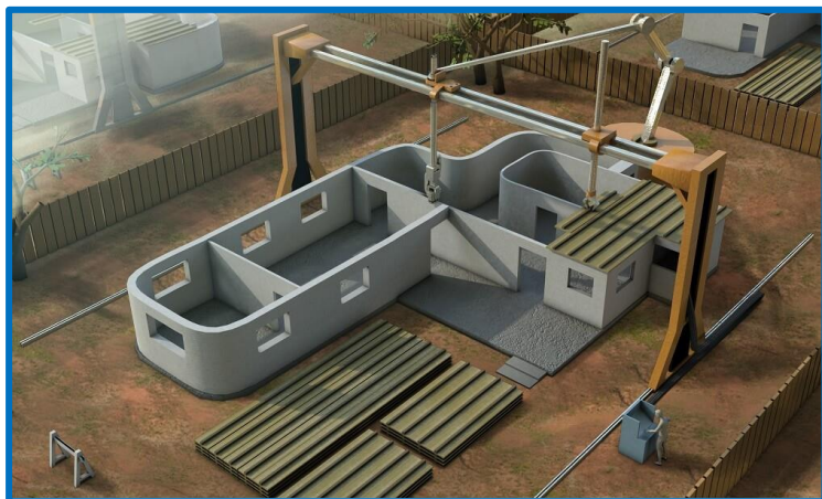
Obrázek 4 - Metoda Contour Crafting [43]
