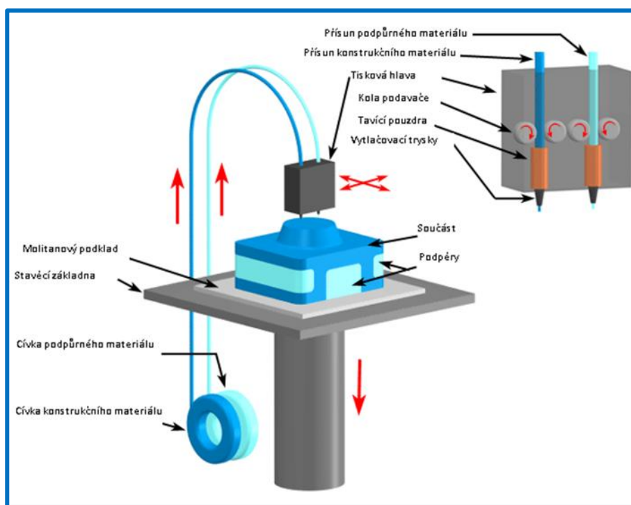
Obrázek 2 - Technologie FDM [42]
