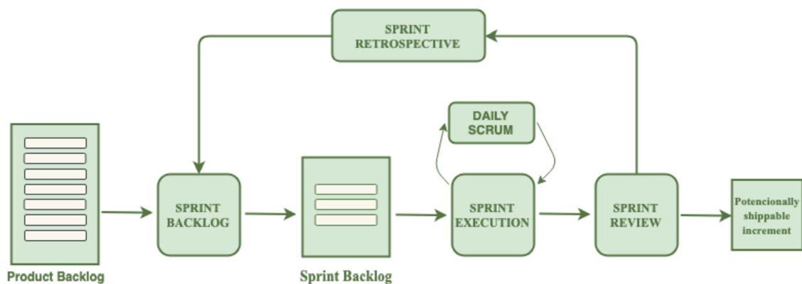
Obrázok 7 Priebeh Scrumu [28]
