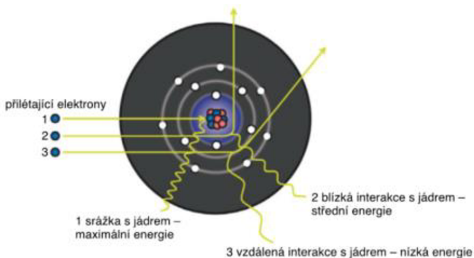
Obrázek 1 – Schematické znázornění vzniku brzdného záření (Zdroj: Malíková et al., 2019)
