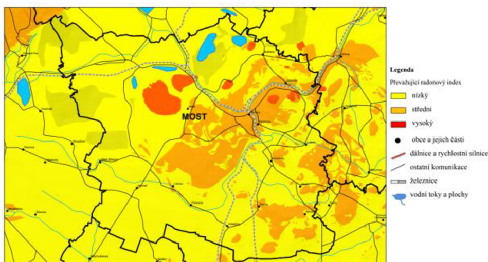
Obrázek 7 – Radonový index na území Mostecka (zdroj: Česká geologická služba)
