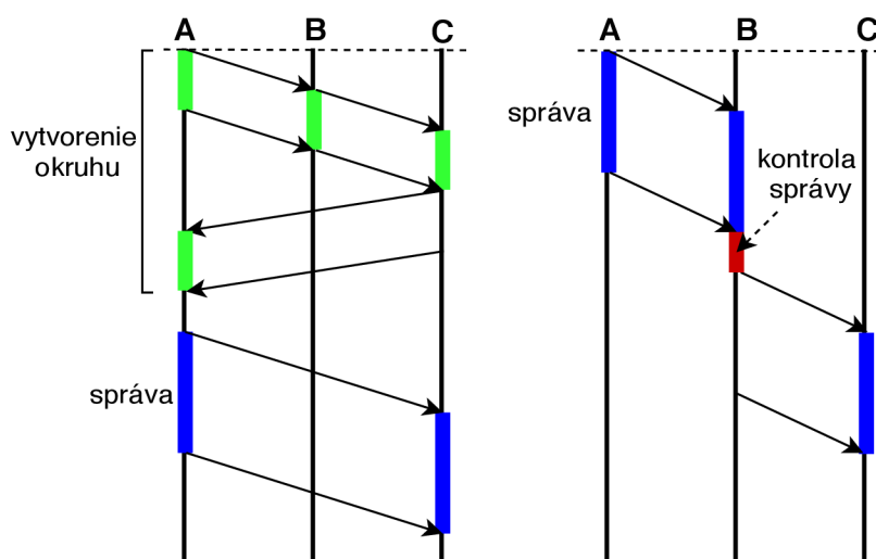
Obr. 3.1: Schéma priebehu prenosu správ pri a) komutácii okruhov, b) komutácii správ [13]
