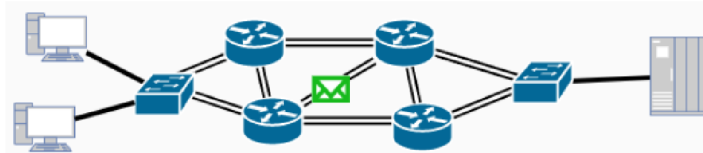
Obr. 9.2: Rezervovanie sieťových prostriedkov pri komutácií okruhov
