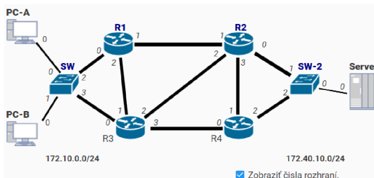
Obr. 9.1: Topológia siete pre simulačný scenár komutácií
