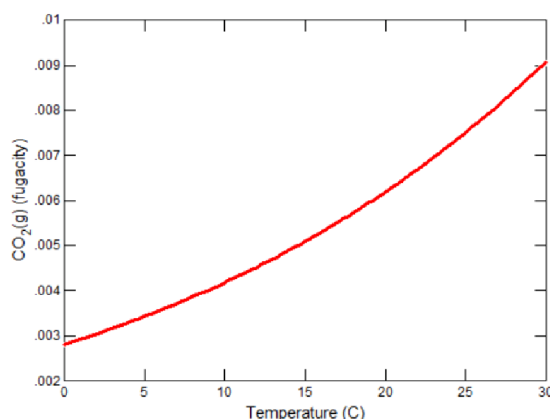
Obrázek 7.2: Fugacita \text{CO}_2 v závislosti na teplotě
