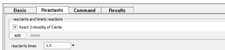
Obrázek 6.3: React - Reactants - Zadání množství postupně přidávaných látek
