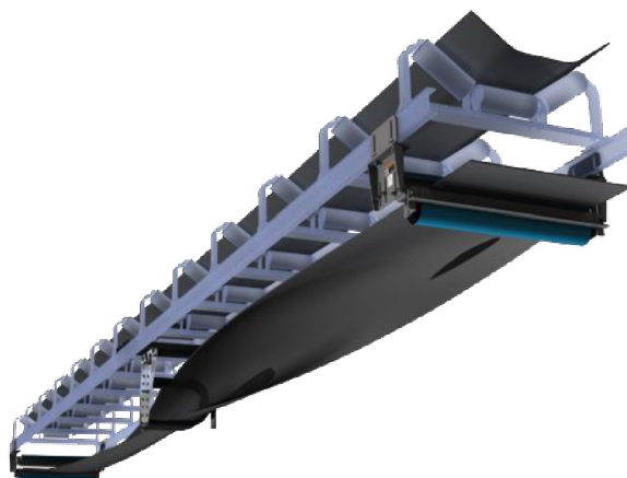
Obrázek 23 Převraceč pásu [39]
