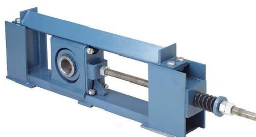
Obrázek 17 Šroubové napínací zařízení [34]
