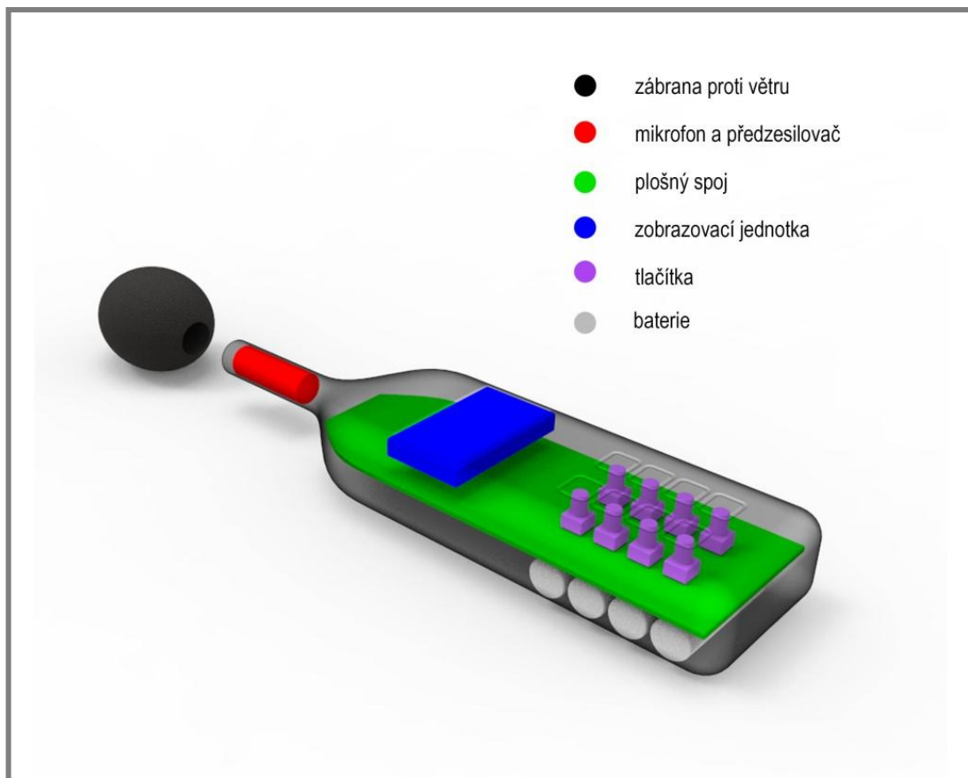
Obr. 2-8 Schéma hlukoměru
