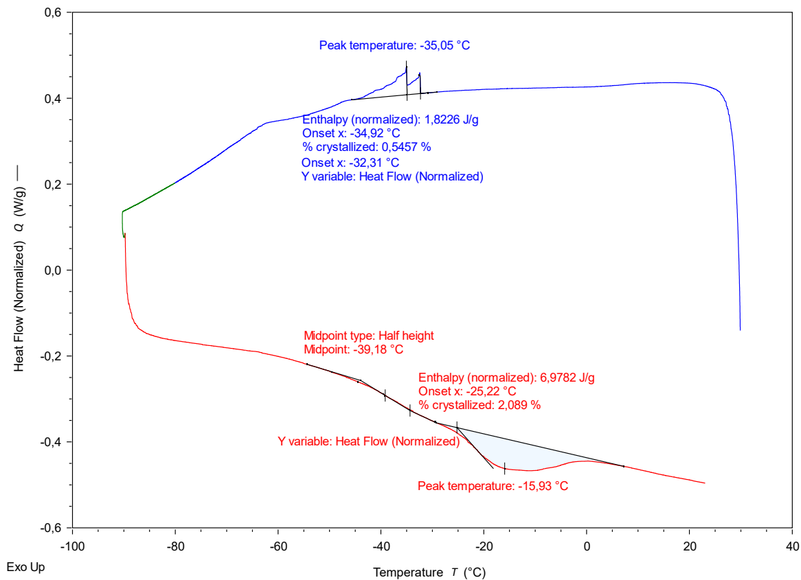
Obrázek F Termogram vzrostných vrcholů chmele, genotyp 14635, izolovaných z kontrolních rostlin po dehydrataci nad silikagelem, při chlazení z teploty +25 °C do -90 °C (modrá křivka) a ohřevu z teploty -90 °C do +25 °C při rychlosti chlazení/ohřevu 10 °C/min. pomocí diferenčního skenovacího kalorimetru Discovery X3 DSC.
