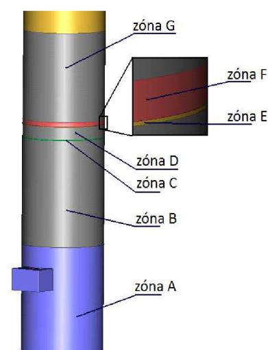
Obr. 9: Vyznačení jednotlivých zón modelu ve výpočtu radiace s UDF.
