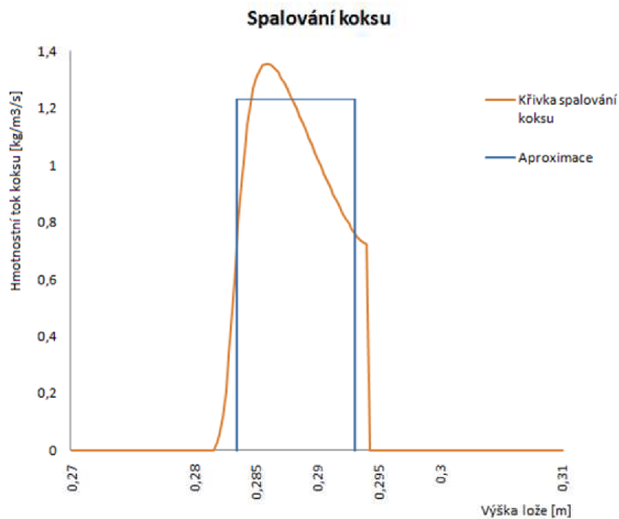
Graf 3: Křivka hmotnostního toku při spalování koksu. Funkční závislost hmotnostního toku koksu [kg/m 3 /s] na výšce lože [m].
