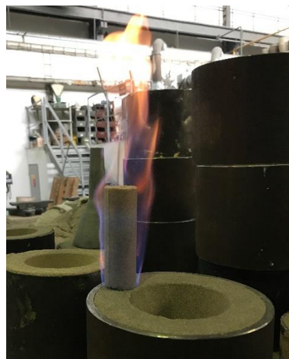
Obr. 36 Vypalování jádra.
