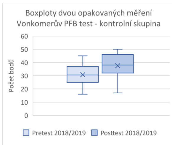
Graf 1: Krabicové grafy výsledku v pretestu a posttestu - kontrolní skupina
