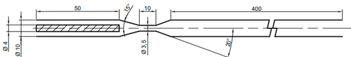
Obrázek 23: Výstupní úhel 20°
