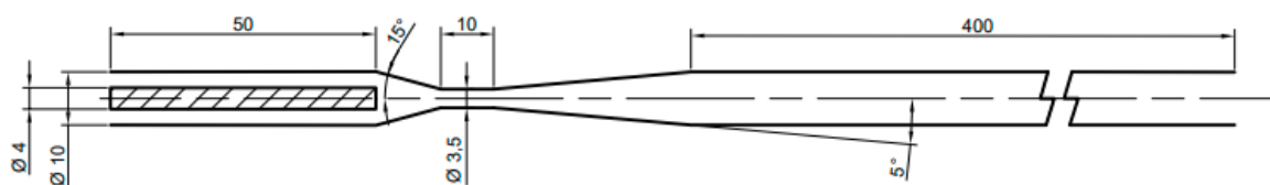
Obrázek 22: Výstupní úhel 5°
