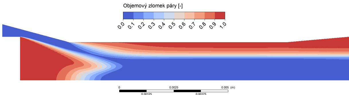
Obrázek 53: Detail kavitace v hrdle trubice
