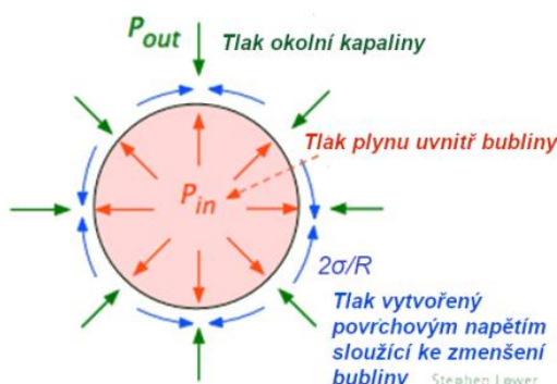
Obrázek 10: Tlak na povrch bubliny v kapalině (upraveno z [42])
