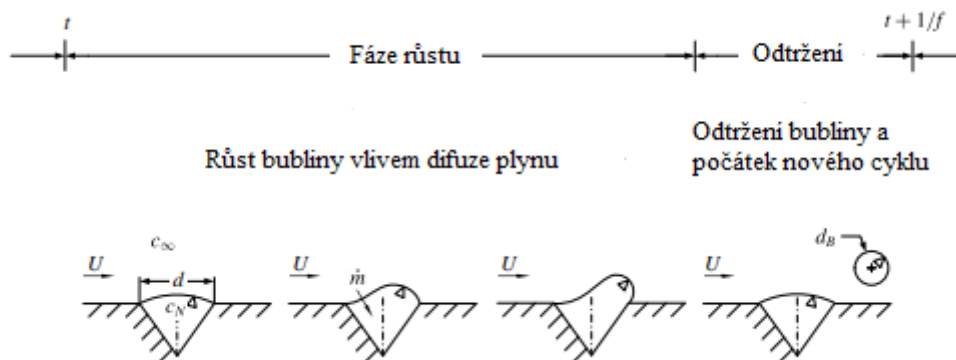
Obrázek 13: Cyklický proces odtrhávání bubliny [39]
