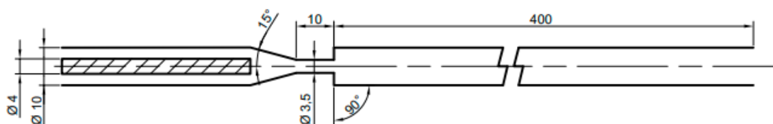
Obrázek 24: Výstupní úhel 90°
