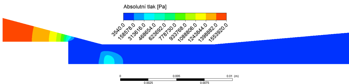
Obrázek 46: Detail tlakového pole v hrdle
