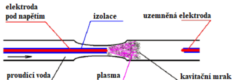
Obrázek 3: Náskres funkční části zařízení CaviPlasma (upraveno z [9])
