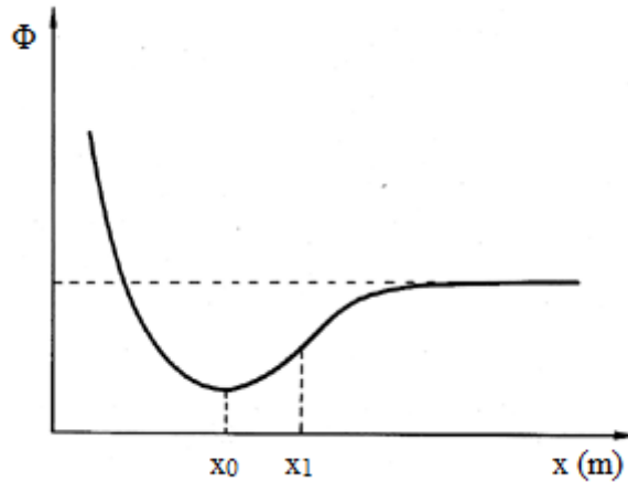
Obrázek 11: Mezimolekulární potenciál [30]
