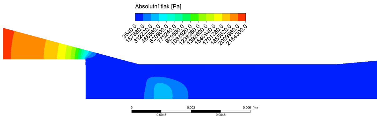
Obrázek 50: Detail tlakového pole v hrdle trubice
