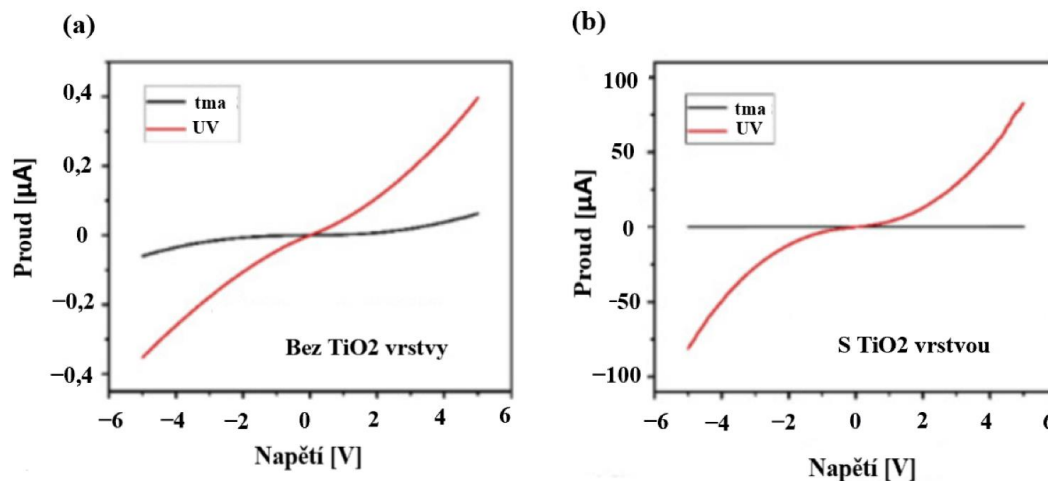
Obr. 6 Voltampérová charakteristika UV detektoru na principu Schottkyho diody (a) bez vložené vrstvy TiO 2 (b) s vrstvou TiO 2 [25]
