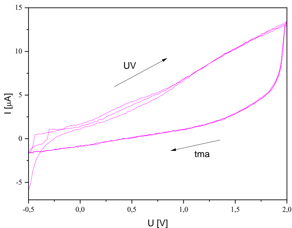
Obr. 22 Cyklická voltametrie UV senzoru se senzorickou vrstvou natištěnou pomocí tamponového tisku a gelovým elektrolytem s 13 % hm. obsahem PVA typ 18-88 vytištěným pomocí sítotisku. Měřeno při intenzitě ozáření 1 \text{ mW/cm}^2 s napětím od -0,5 do 2 \text{ V}
