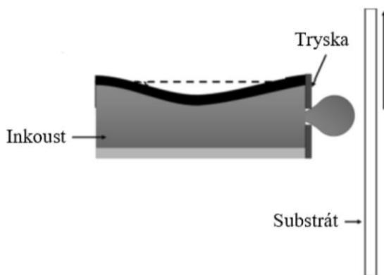
Obr. 3 Schéma fungování piezelektrické inkoustové tiskárny [17]
