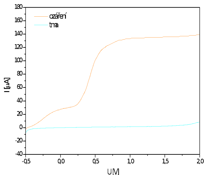
Obr. 10 Ukázka voltamperové charakteristiky fotoelektrochemického senzoru sintrované elektrody s kapalným elektrolytem. Sensorická vrstva TiO 2 byla natištěna na FTO sklo. Jako elektrolyt byl použit kapalným roztok 0,1 M H 2 SO 4 . Měřeno při intenzitě ozáření 1 mW/cm 2 s napětím od -0,5 do 2 V [42]
