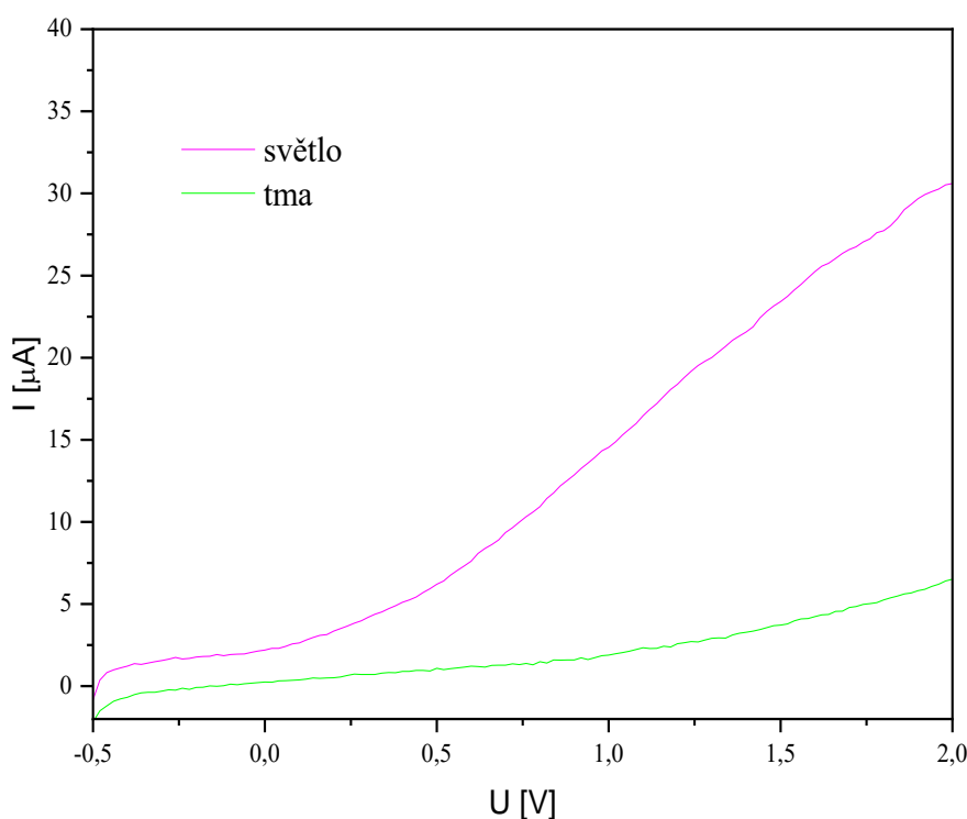
Obr. 21 Lineární voltametrie UV senzoru se sensorickou vrstvou natištěnou inkoustovým tiskem a 13 % hm. obsahem PVA typu 18-88. Vzorek měřen za intenzity ozáření 1\text{mW/cm}^2 s napětím v rozmezí od -0,5 do 2\text{ V}
