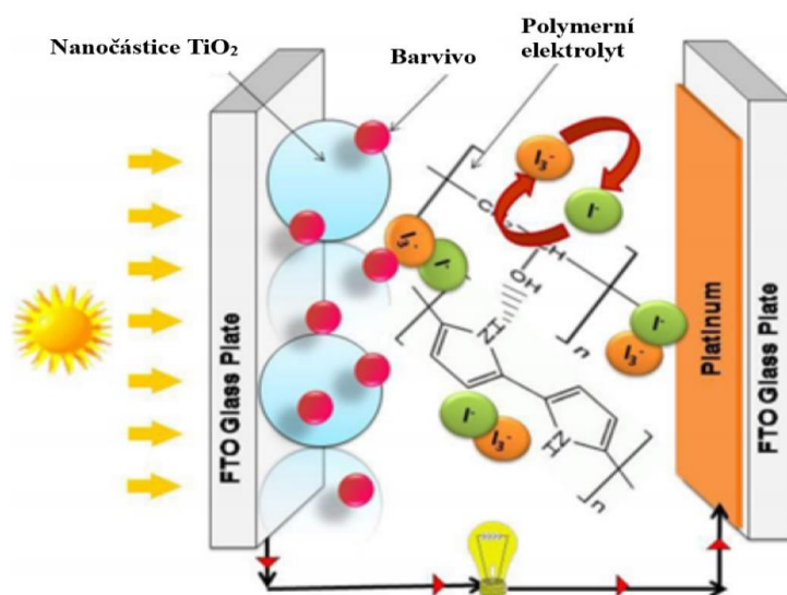
Obr. 8 Schéma vodivého polymerního elektrolytu pro konstrukci barvivem senzibilizovaných solárních článků s kombinací PVA, PPy a redoxního páru KI/I 2 [31]
