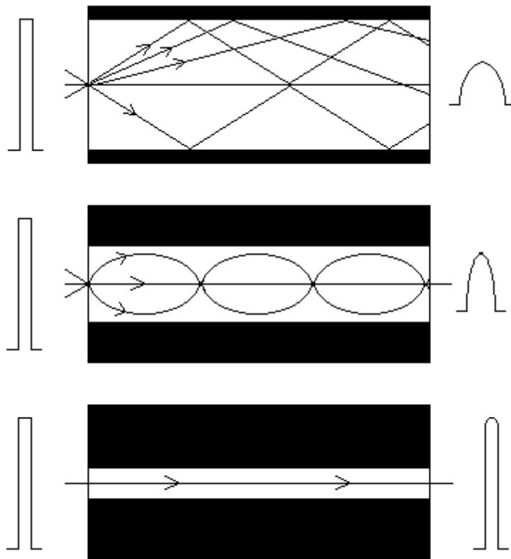
Obr. 4.1: Šíření impulzů vláknem (Mnohovidové vlákno se skokovou změnou indexu lomu, mnohovidové vlákno gradientní, jednovidové vlákno se skokovou změnou indexu lomu) [2]
