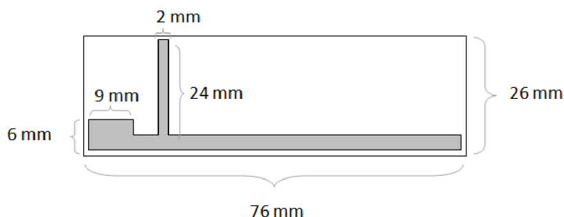
Obr. 23: Návrh katody (šedá oblast znázorňuje Au, bílá korundová destička)
