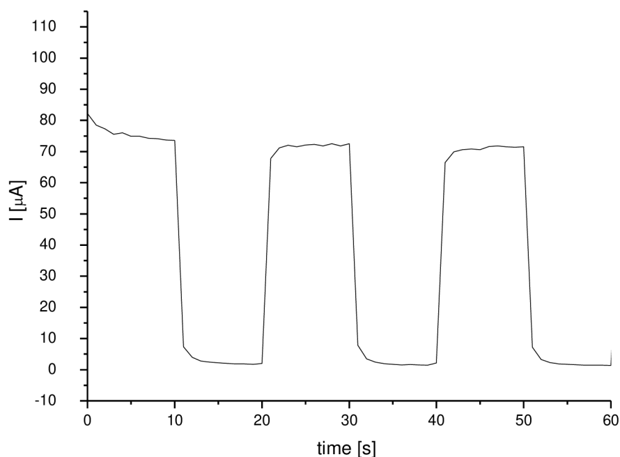
Obr. 8: Ukázka chronoamperometrického měření (záznam generovaného proudu při vkládání konsistentního napětí 1 V v závislosti na čase při střídání měření s UV ozářením a bez ozáření v trvání 10 s)
