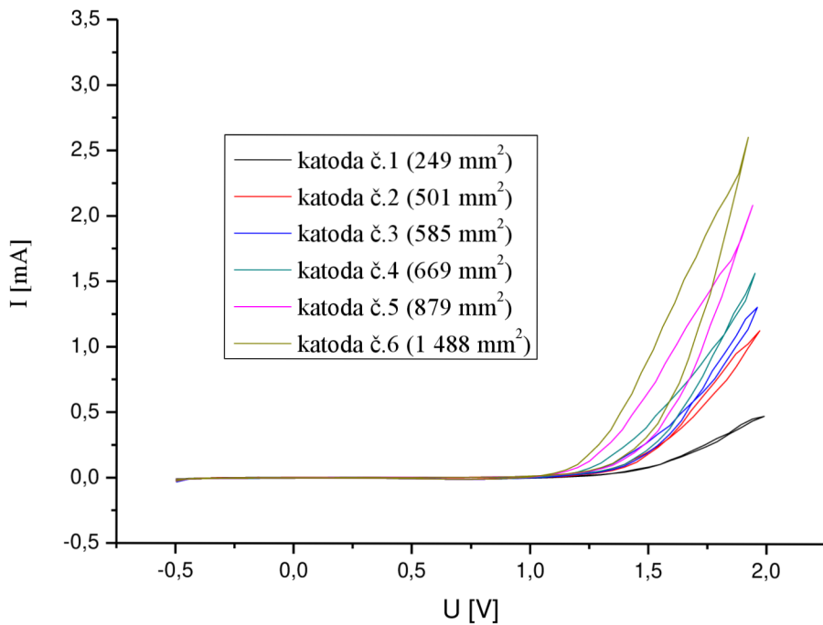
Obr. 34: Temnostní křivka lineární voltametrie (porovnání různých ploch protielektrod)
