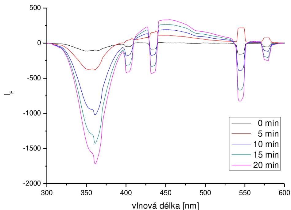
Obr. 14: Emisní spektrum reakční směsi degradace kyseliny benzoové v závislosti na čase reakce ( c_{BA}=1 \cdot 10^{-3} \text{ mol/dm}^3 , elektrofotokatalytický režim s přepětím)
