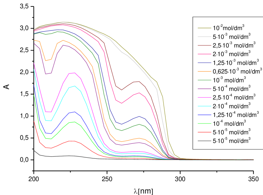
Obr. 18: Absorpční spektrum kyseliny benzoové o různých koncentracích [42]
