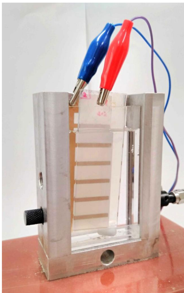
Obr. 12: Ukázka kyvety pro měření fluorescence
