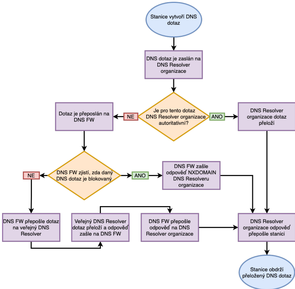
Obr. 3.1: Zasazení DNS firewallu do systému vyhodnocení DNS dotazu
