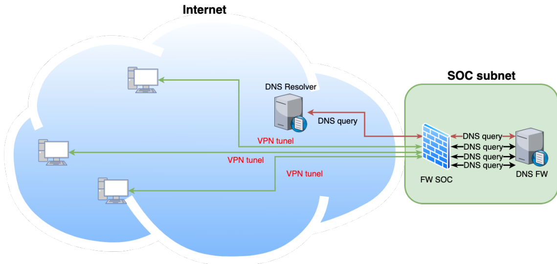
Obr. 5.4: Napojení koncových stanic na DNS FW pomocí VPN
