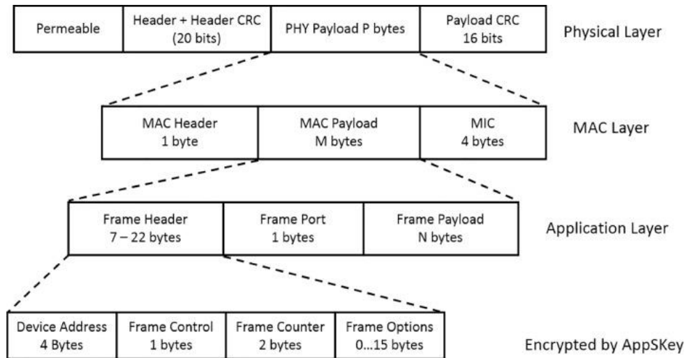
Obr. 11. Datový rámeček LoRaWAN [18]
