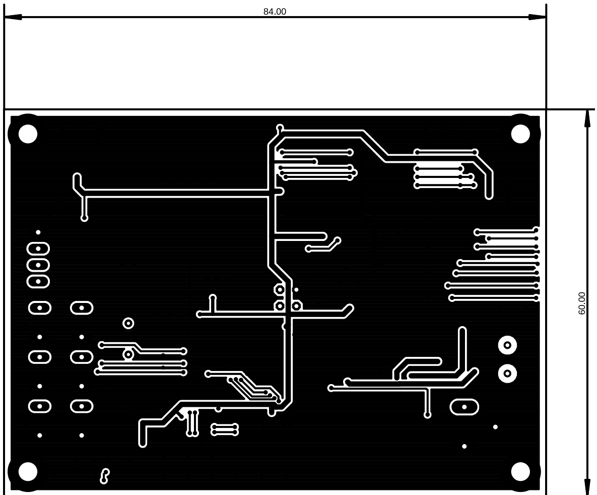
Obr. B2. Okótovaný DPS motiv ze spodní strany
