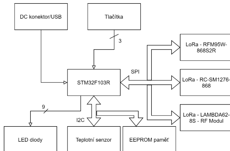
Obr. 14. Blokové schéma koncového zařízení
